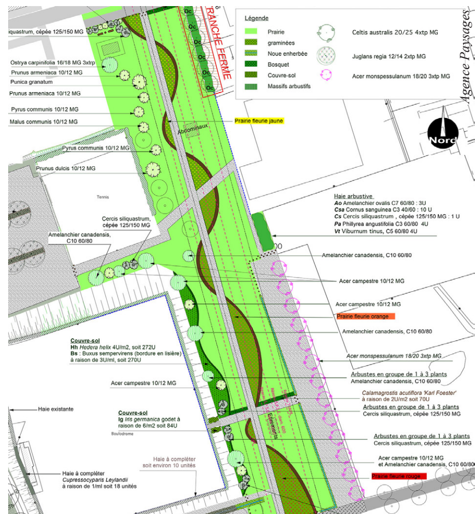
Fig. 25 : Extrait du plan de plantations de l'axe pipelines du Quartier Queue Longue Nord
