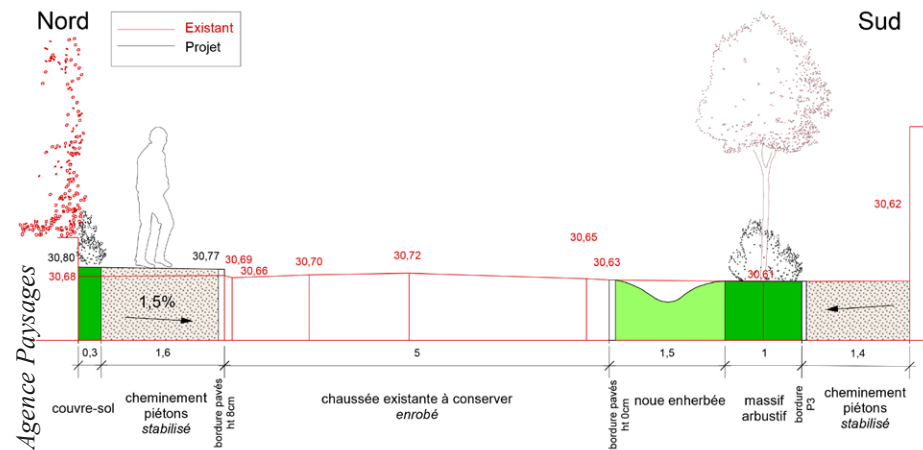
Fig. 19 : Profil en travers du projet de l'avenue Jean Moulin
