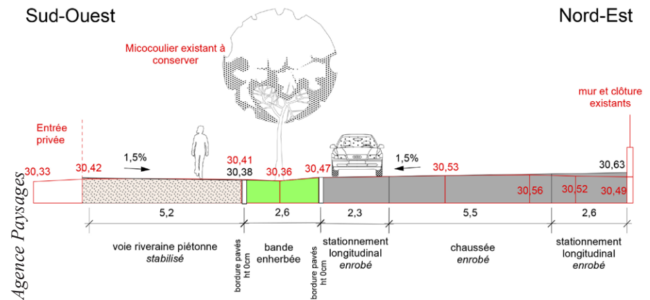
Fig. 21 : Profil en travers du projet de la rue Gaston Ferrié
