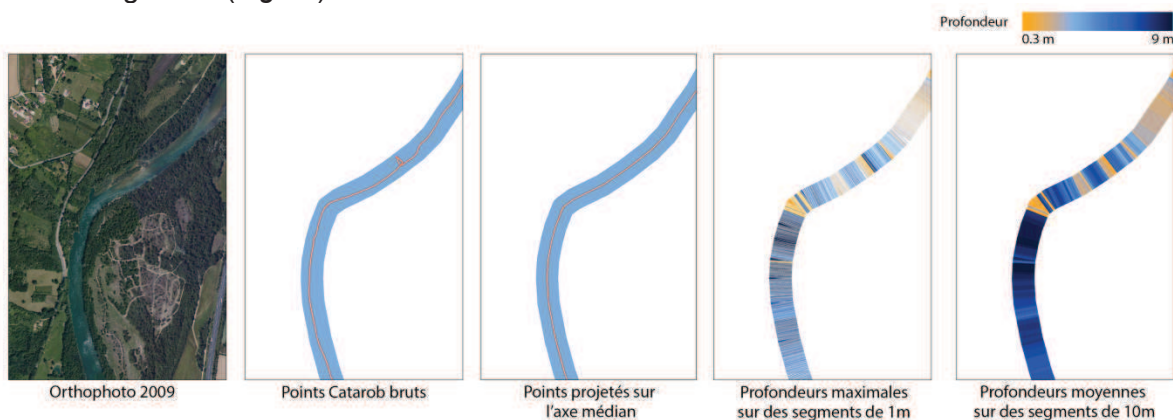
Figure 30 : Principales étapes de lissage du profil en long (Extrait aux PK 4000 à 5600)
