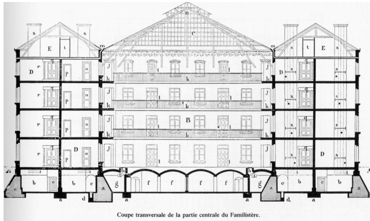
Coupe transversale de la partie centrale du Familistère.
