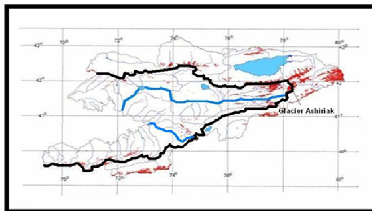
Figure 3 : Localisation du bassin versant du Syr Daria au Kyrgyzstan (intérieur de la courbe noire) avec localisation des glaciers (en rouge) (©UNDP, 2009)
