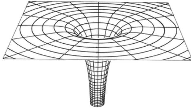
Illustration 10. Représentation géodésique de l'espace-temps déformé par un trou noir
