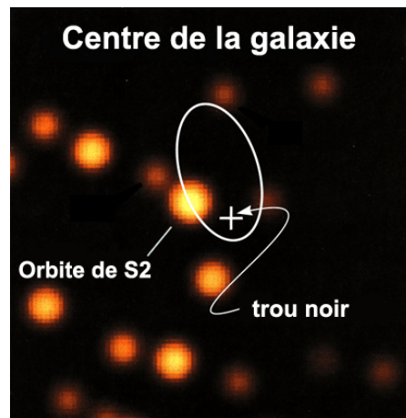
Illustration 17. Mise en évidence de Sagittarius A via l'orbite de l'étoile S2 par l'équipe d'Andrea Ghez
