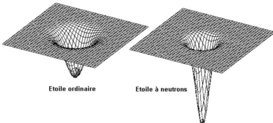
Illustration 12. Modélisation géodésique du champ d'attraction de deux astres
