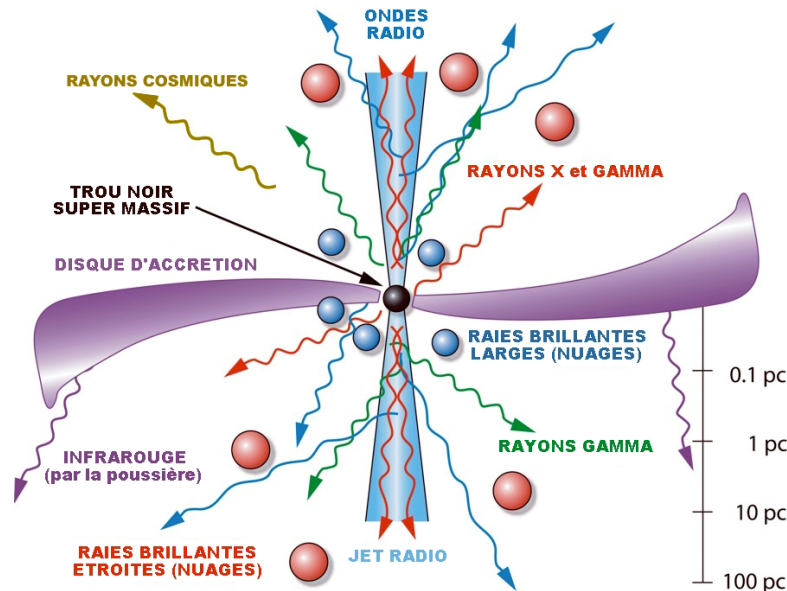
Illustration 13. Représentation schématique des rayonnements induits par la présence d'un trou noir
