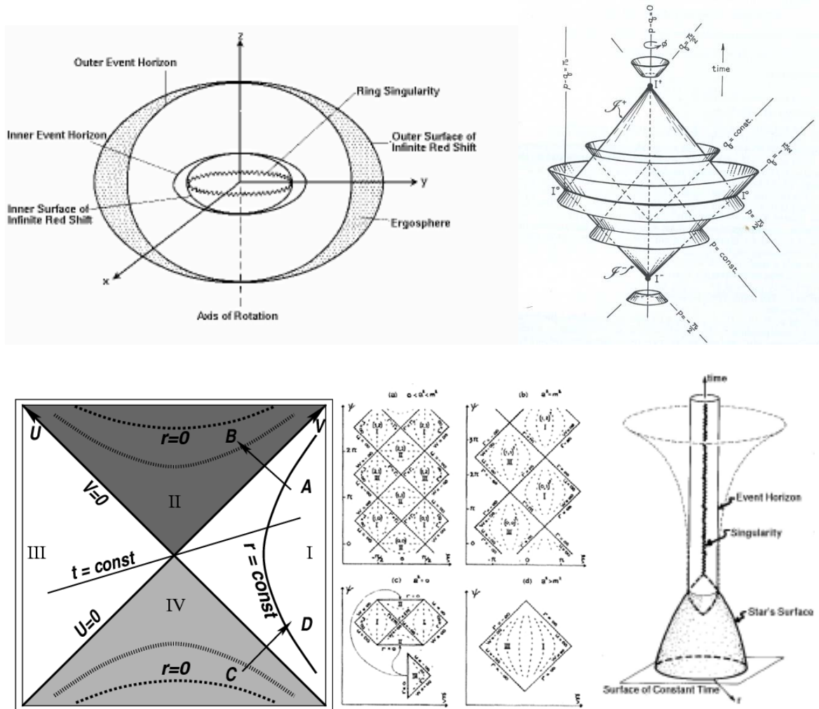
Illustration 9. Représentations schématiques de trous noirs
