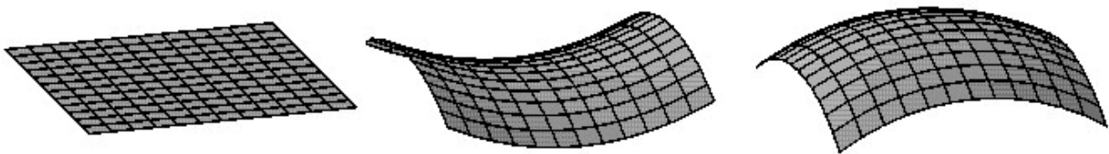
Illustration 11. Modélisation des courbures de l'espace.
