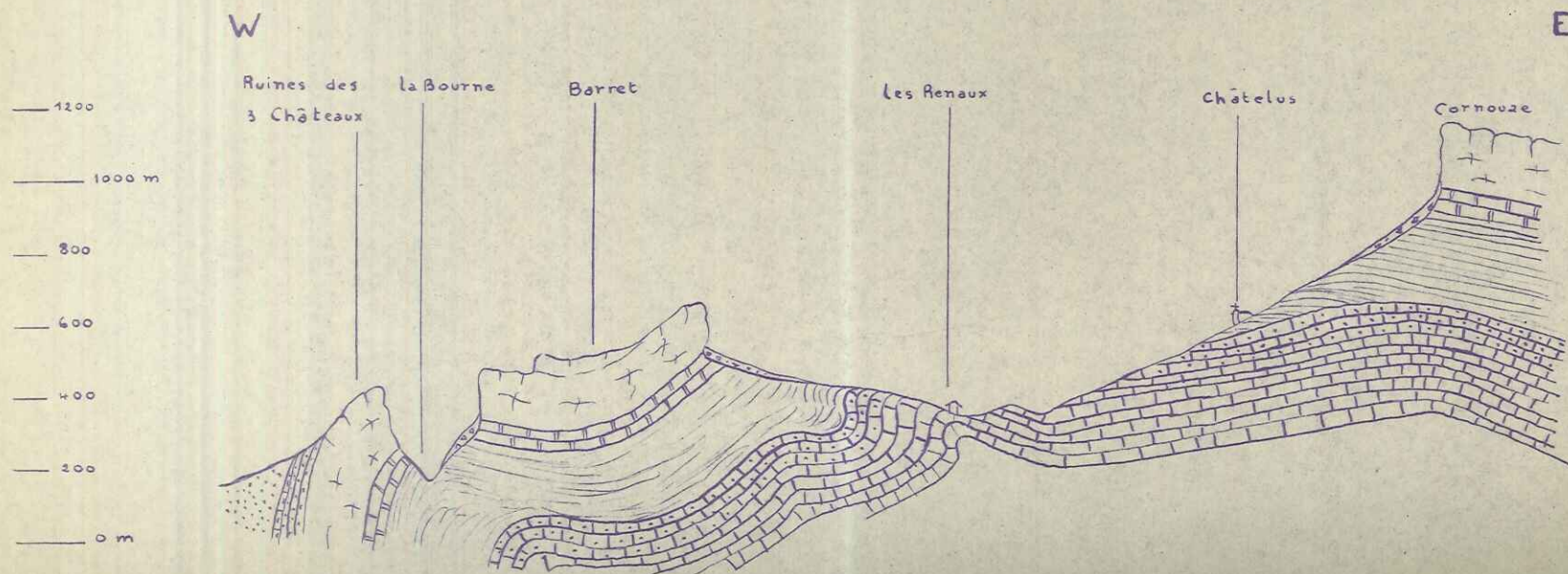
Coupe n°3
