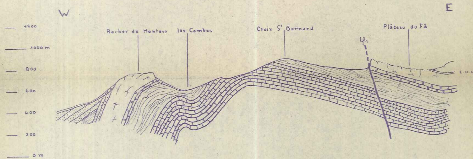
Coupe n° 10
