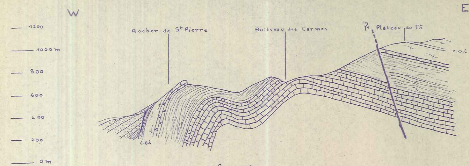
Coupe n° 12
