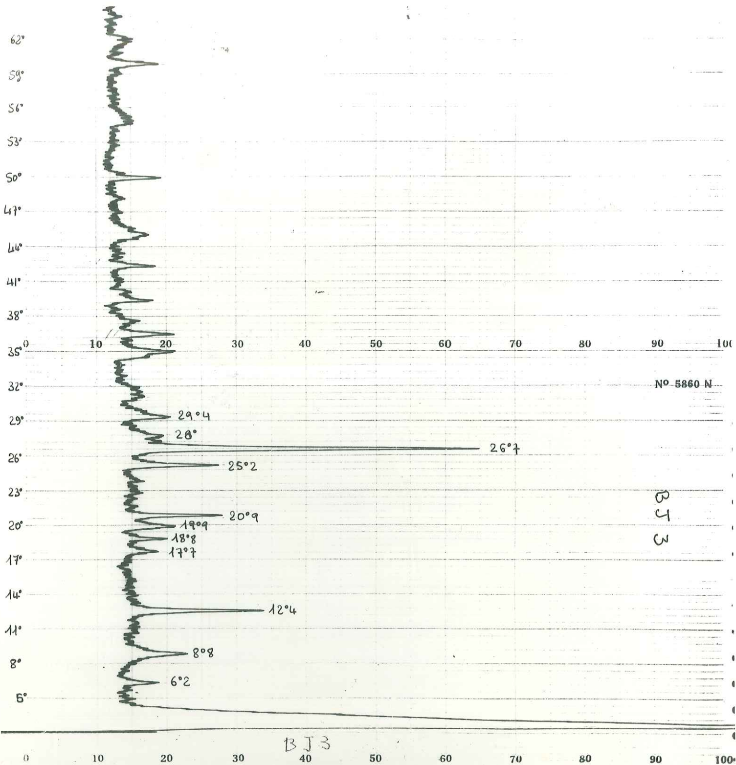
SPECTRE DE DIFFRACTION X (POUDRES) MARNES BAJOCIENNES
