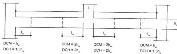
FIG. 2.12 — Étendues des zones critiques dans les poutres.
