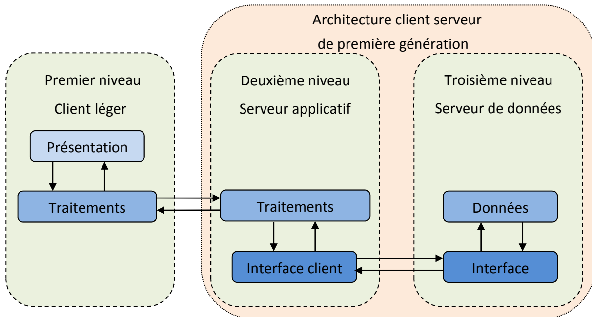
Figure 21 : Schéma d'une architecture 3-tiers
