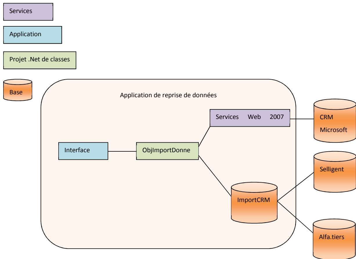
Figure 10 : Schéma simplifié du logiciel de reprise de données
