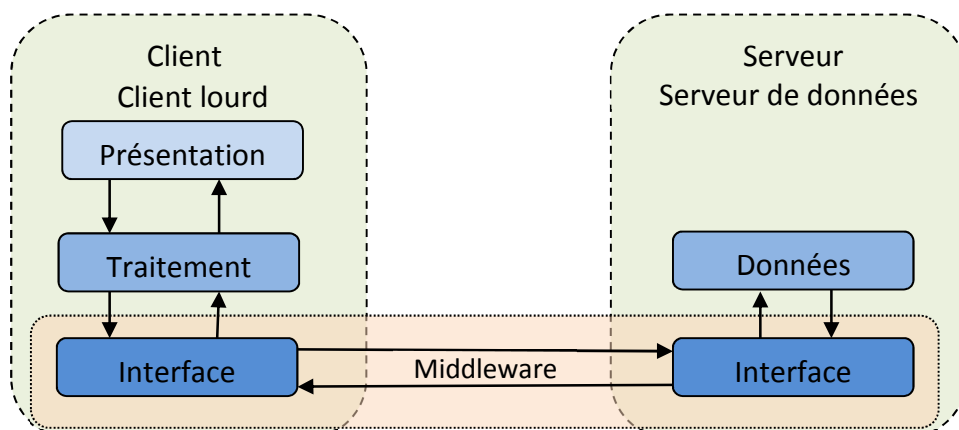
Figure 20 : Schéma d'une architecture client-serveur
