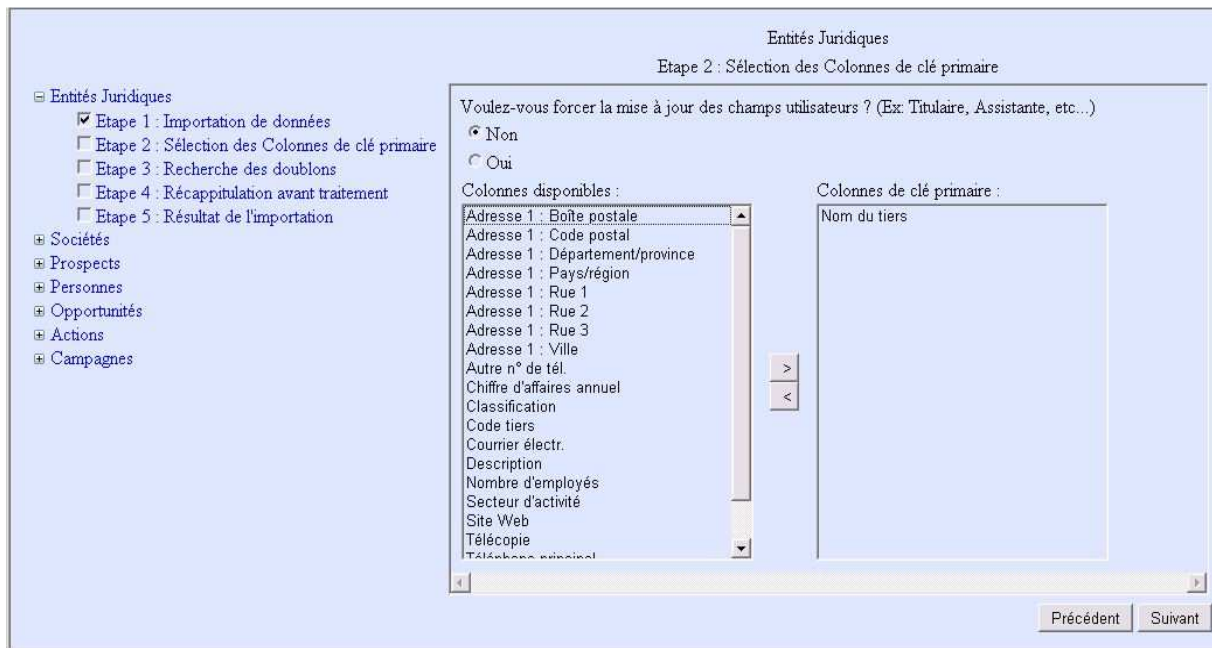
Figure 12 : Etape 2 - Sélection des colonnes de clé primaire
