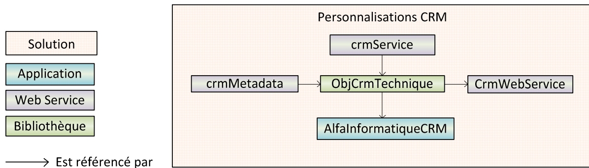
Figure 9 : Nouvelle organisation des projets au sein de la solution des personnalisations du logiciel de CRM
