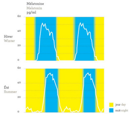
Variation du taux de Mélatonine dans le sang en fonction de la variation de la luminosité solaire. Variation of rate of melatonin in blood in phase with variation of sunlight. Sources: Décoaster & Rabier - Architecture Physiologique - ed. Birkhäuser
