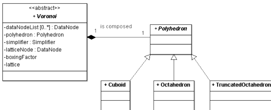
FIGURE 2.11 – Diagramme de classe de la gestion des Voronoi s.
