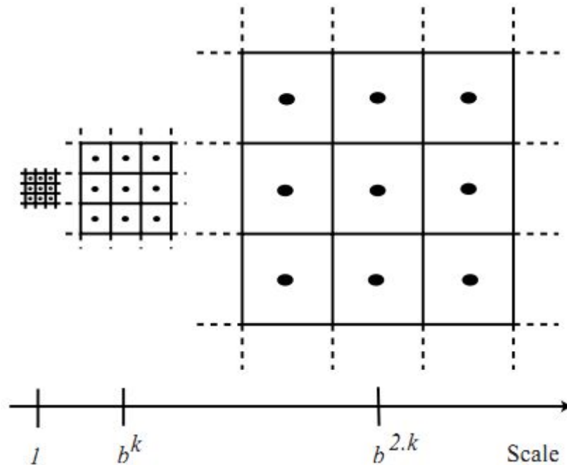
FIGURE 1.25 – Hiérarchie de réseaux cubiques en 2D. Facteur d'échelle b=3
