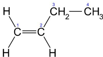
FIGURE 1.7 – Formule développée plane du 1-butène ( \text{C}_4\text{H}_8 ).
