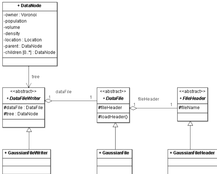
FIGURE 2.15 – Diagramme de classe de l'export de données (écriture de fichier cube ).
