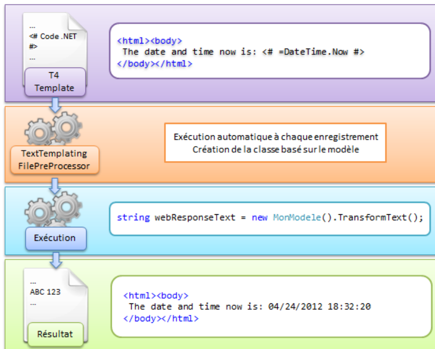
Figure 25 - Processus de génération avec un modèle T4 "Run Time"
