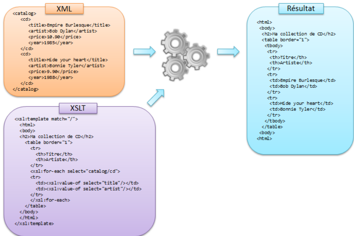
Figure 29 - Exemple d'une transformation XSLT
