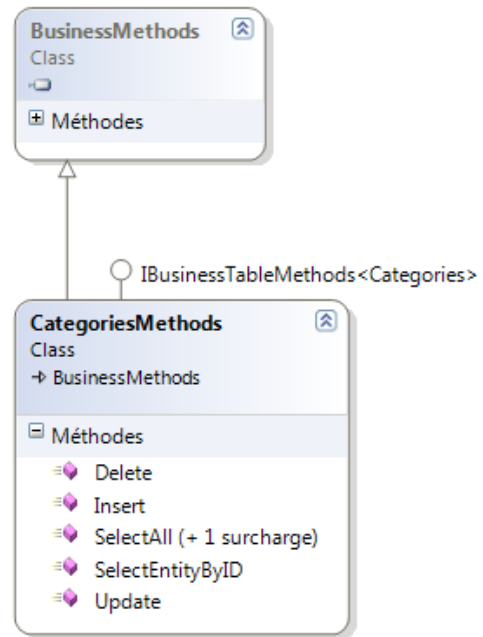
Figure 53 - Diagramme de classes - Exemple de classe "méthodes" générée
