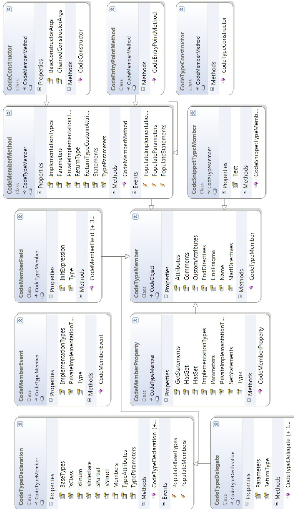
Figure 72 - Détails de la classe CodeType
