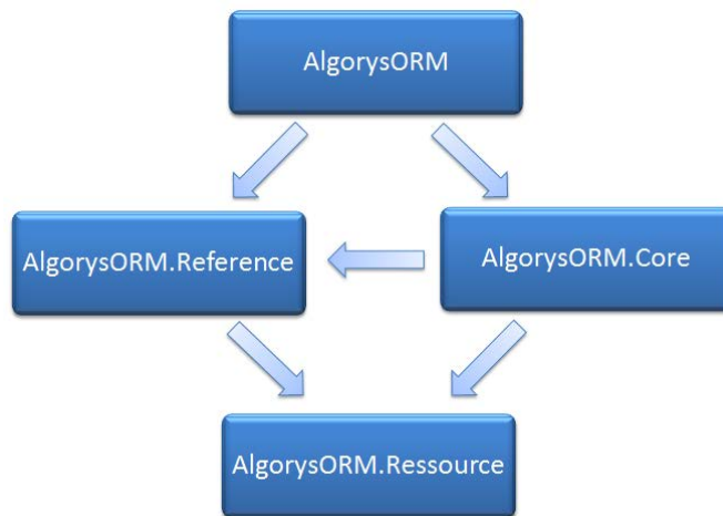
Figure 46 - Dépendances des bibliothèques AlgorysORM
