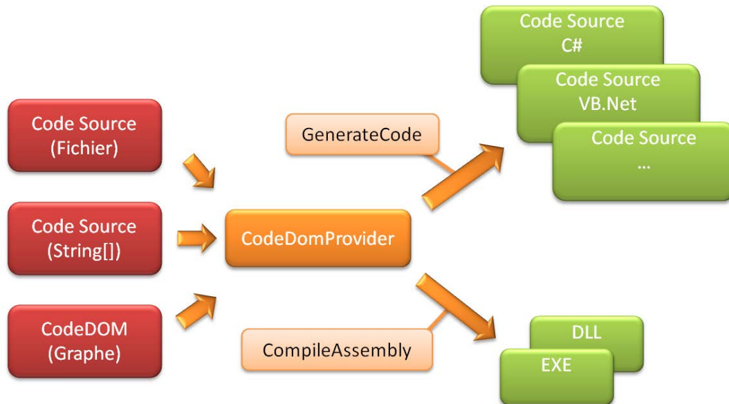
Figure 30 - Schéma de principe CodeDOM
