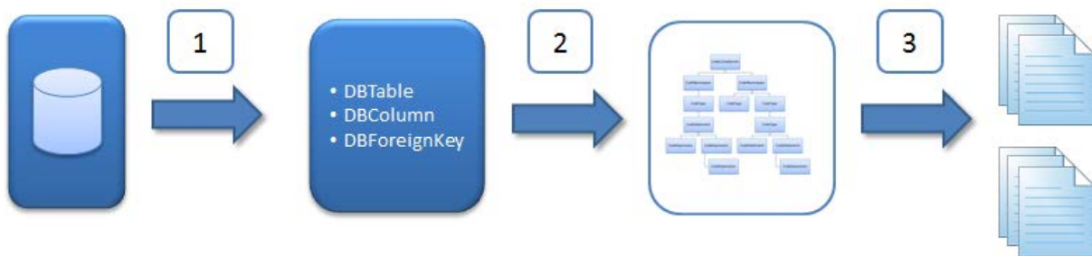
Figure 49 - Schéma de génération de la couche ORM
