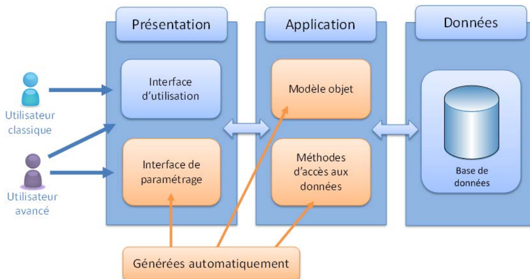
Figure 7 - Définition des modules à générer
