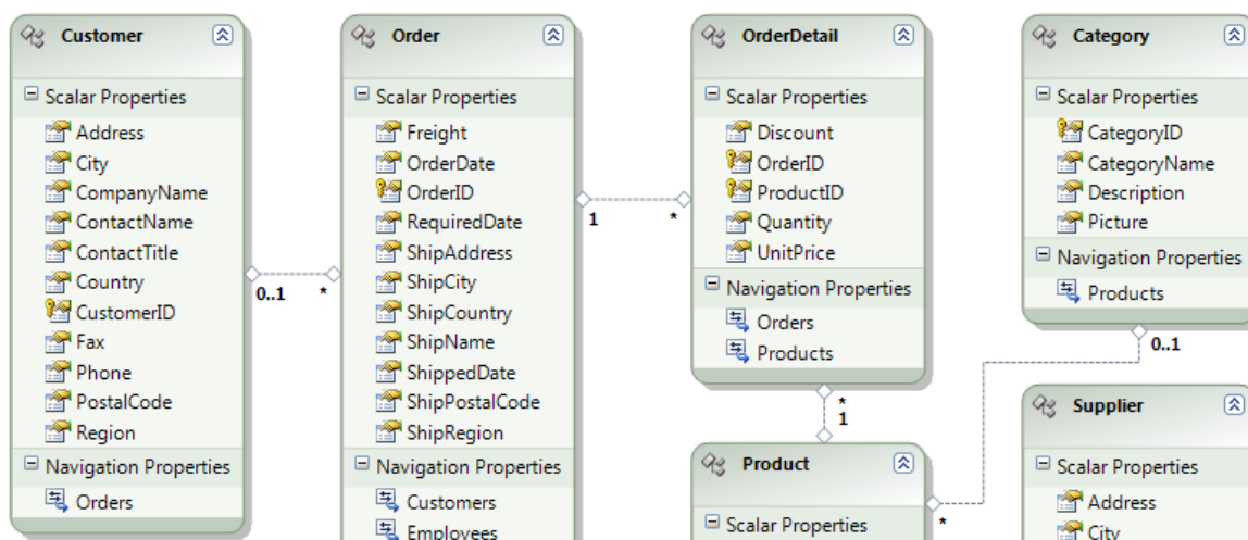
Figure 18 - Exemple de schéma conceptuel sous Visual Studio
