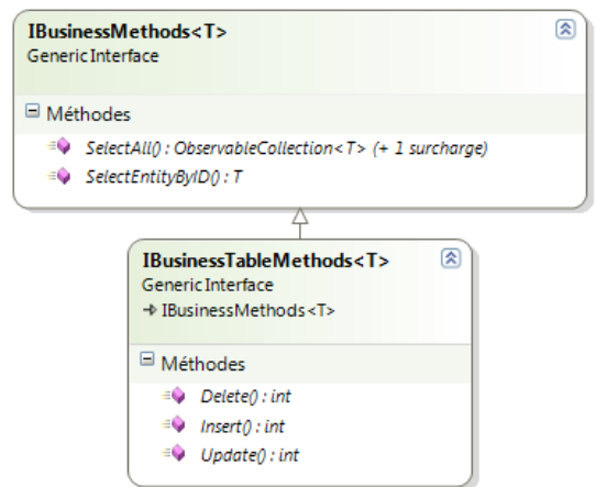
Figure 55 - Diagramme de classes - Interfaces pour les classes "méthodes"
