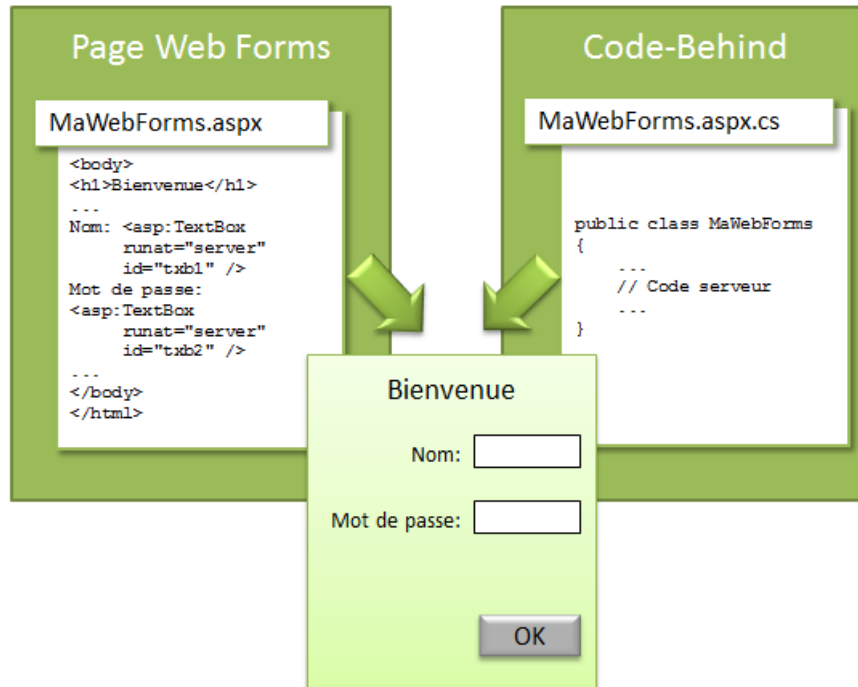
Figure 44 - Web Forms : Structure des fichiers
