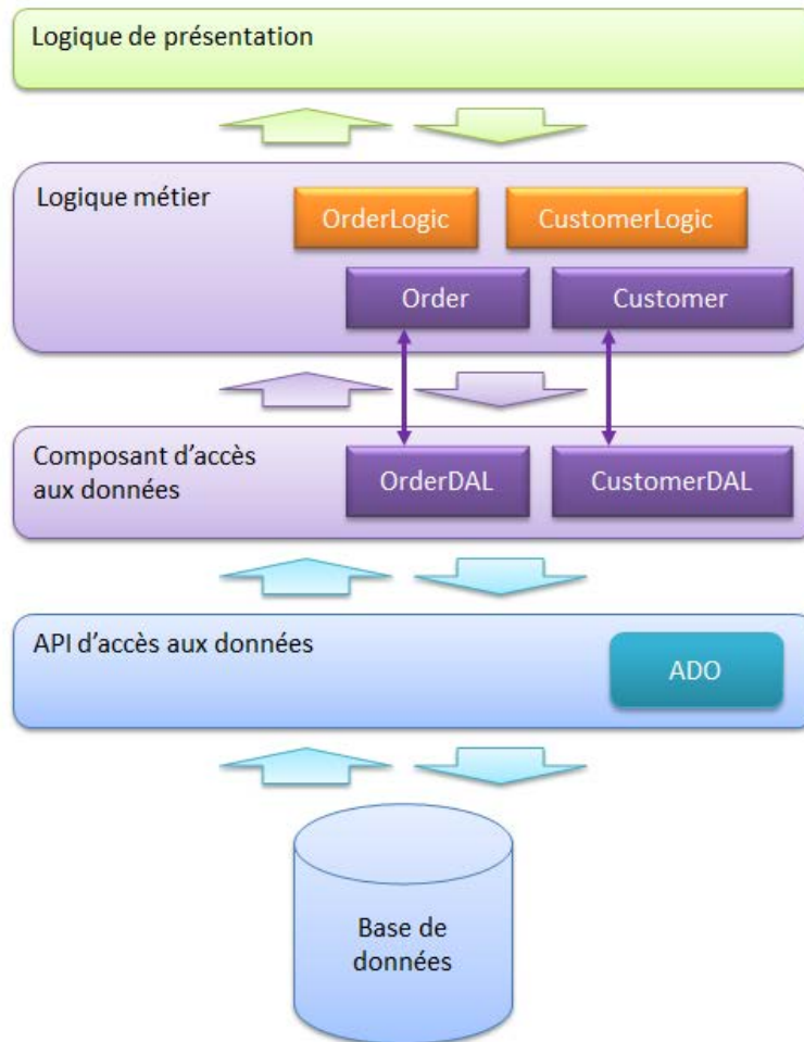
Figure 12 - Architecture de référence
