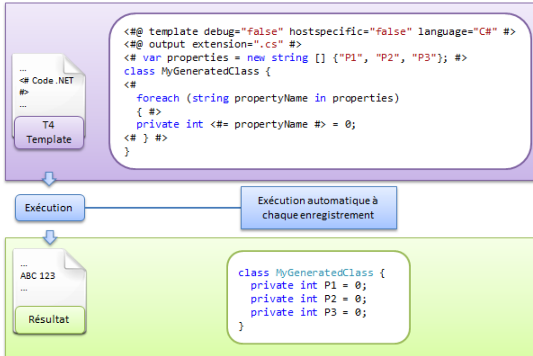
Figure 27 - Processus de génération d'un modèle T4 "Design Time"
