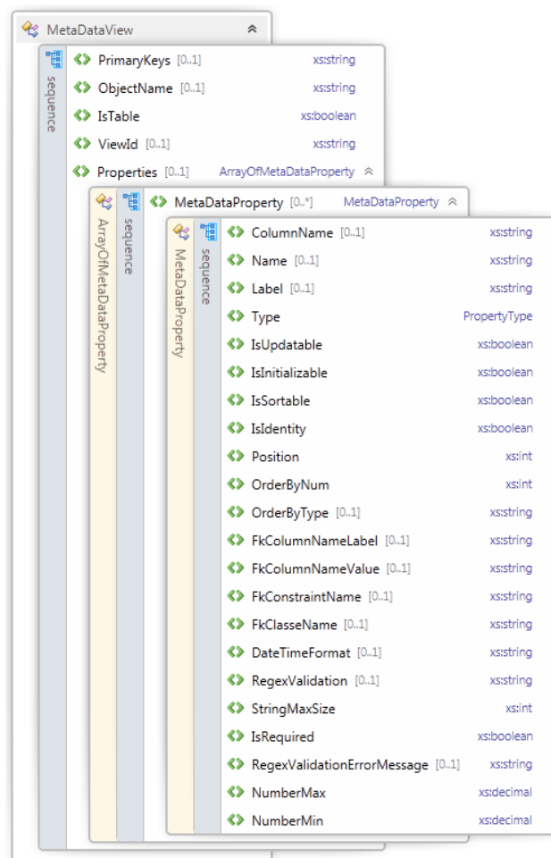
Figure 42 - Détail du schéma XML des métadonnées – MetaDataColumn
