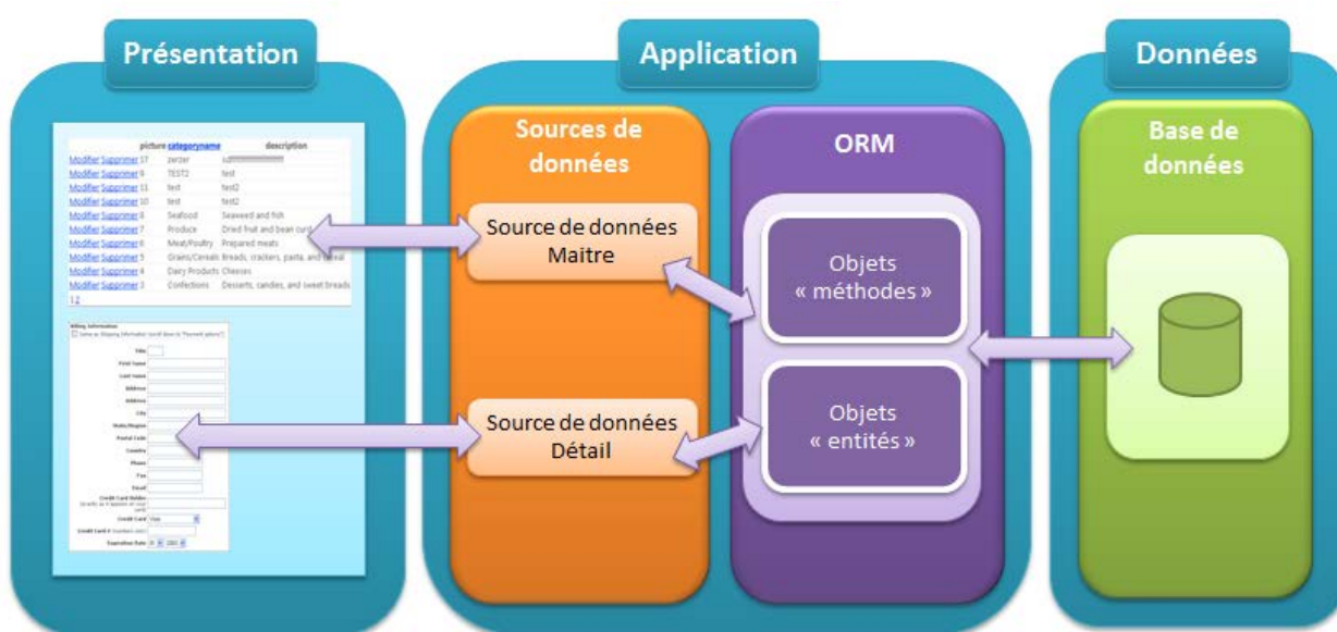
Figure 57 - Schéma de principe de l'architecture du composant
