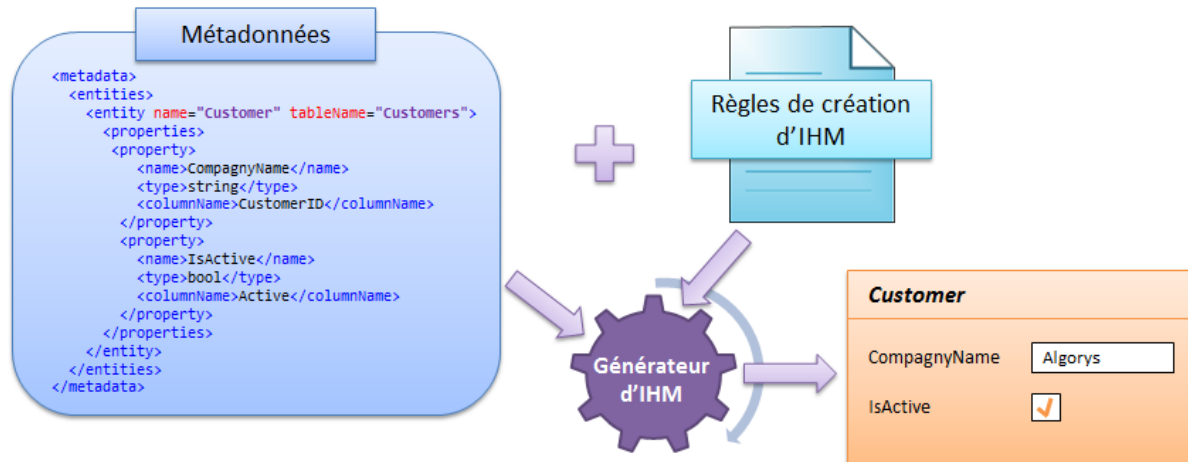
Figure 39 - Exemple de génération d'IHM
