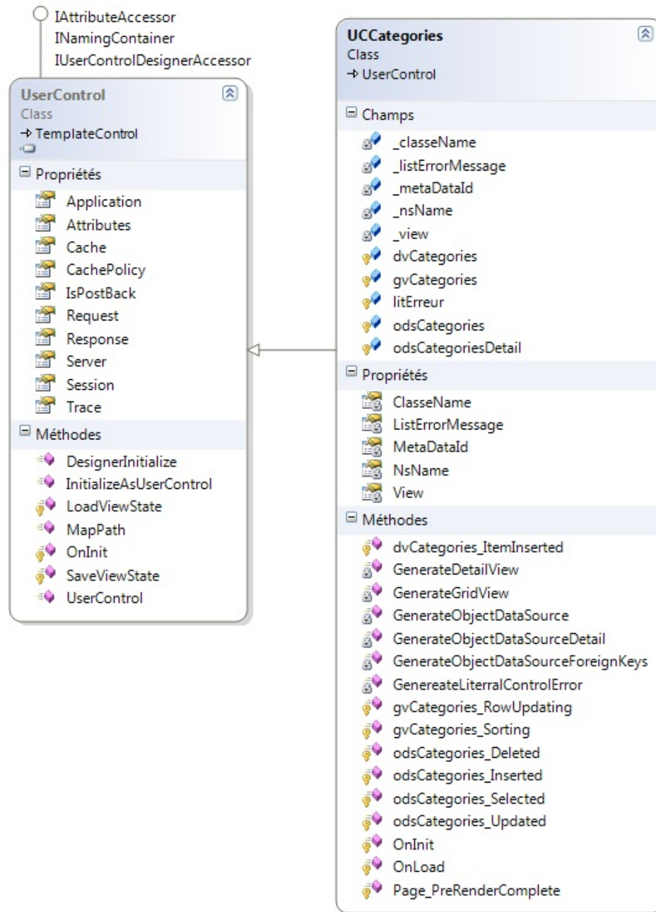
Figure 63 - Diagramme de classes - Exemple d'une classe correspondant à une table Categories
