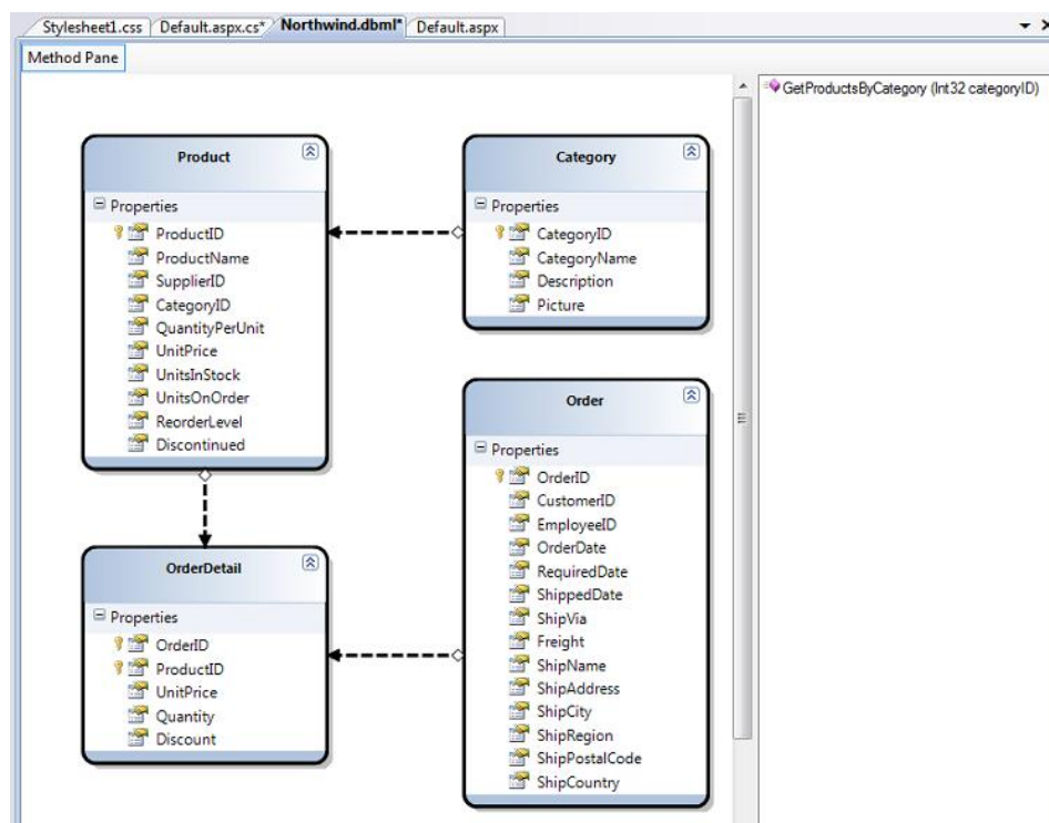
Figure 13 - Concepteur de modèle LINQ to SQL 1
