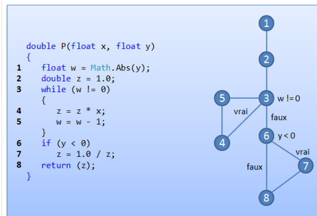
Figure 65 - Diagramme de flux de contrôle
