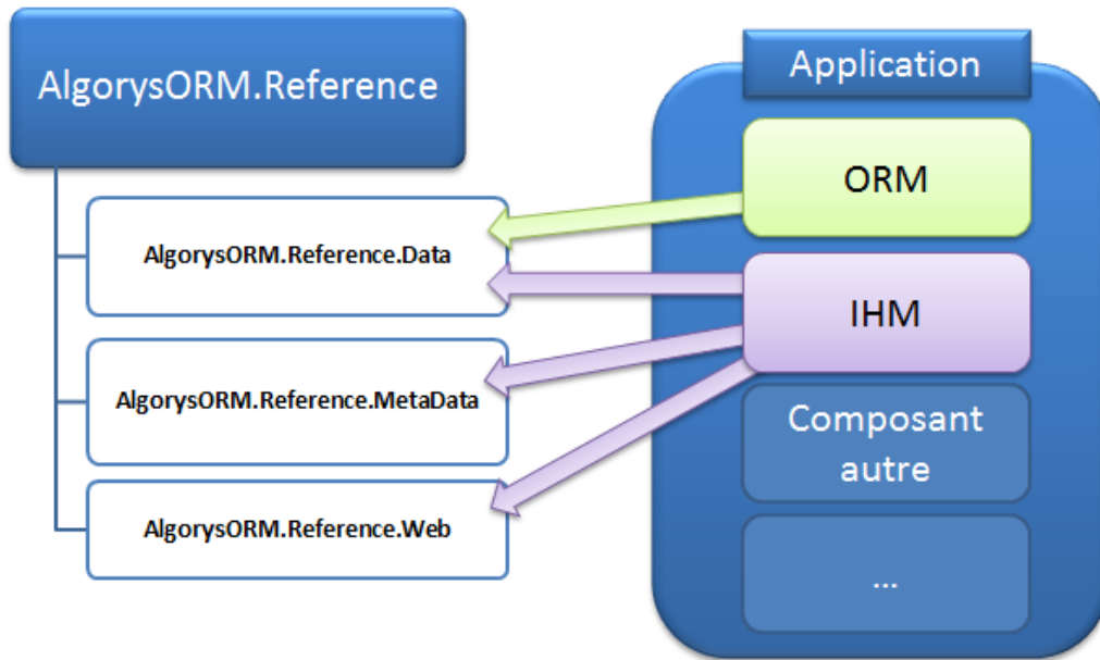
Figure 47 - Schéma de référencement entre l'application et la bibliothèque logicielle AlgorysORM.Reference
