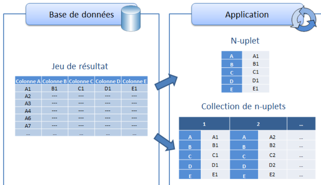
Figure 11 - Schéma de l'approche n-uplet
