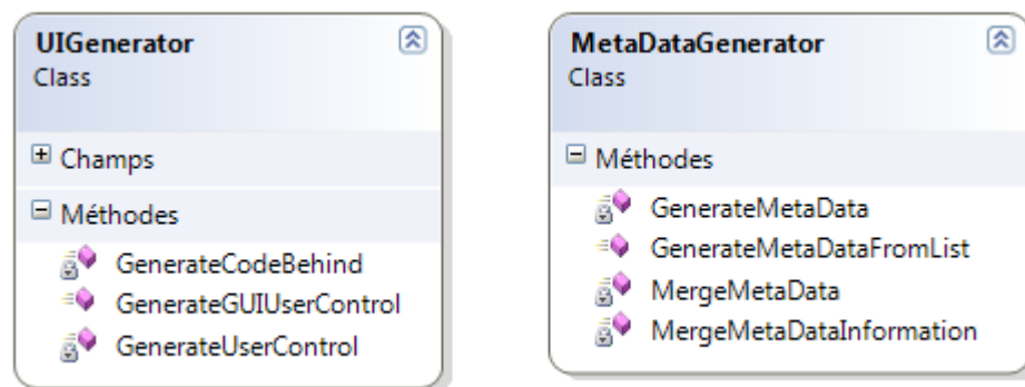
Figure 61 - Diagramme de classes – Génération du code source pour le formulaire
