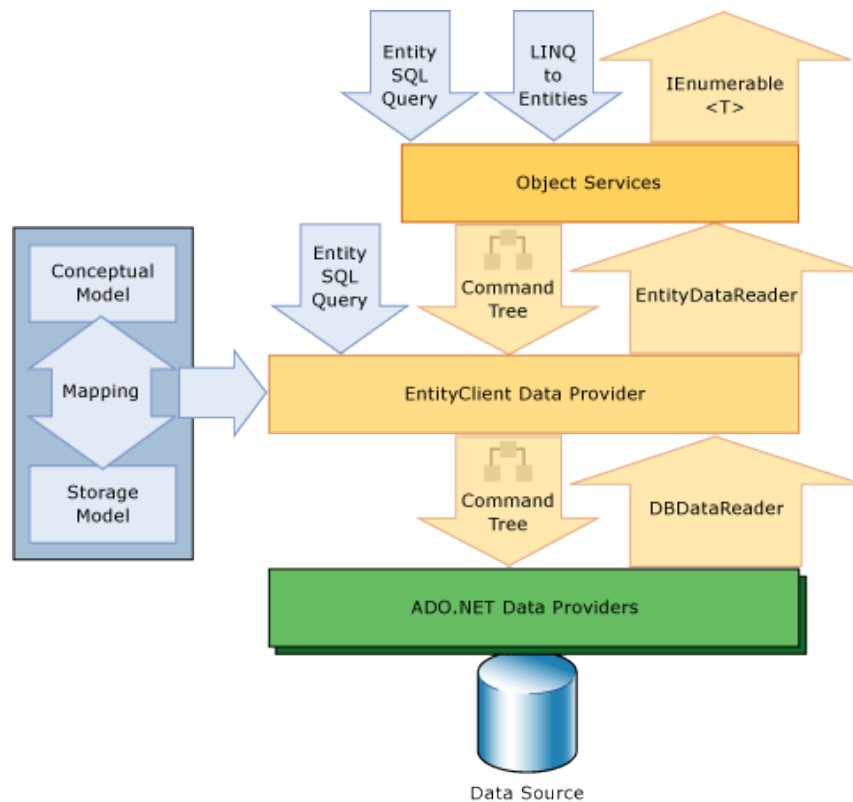
Figure 19 - Schémas d'interrogation des données dans Entity Framework
