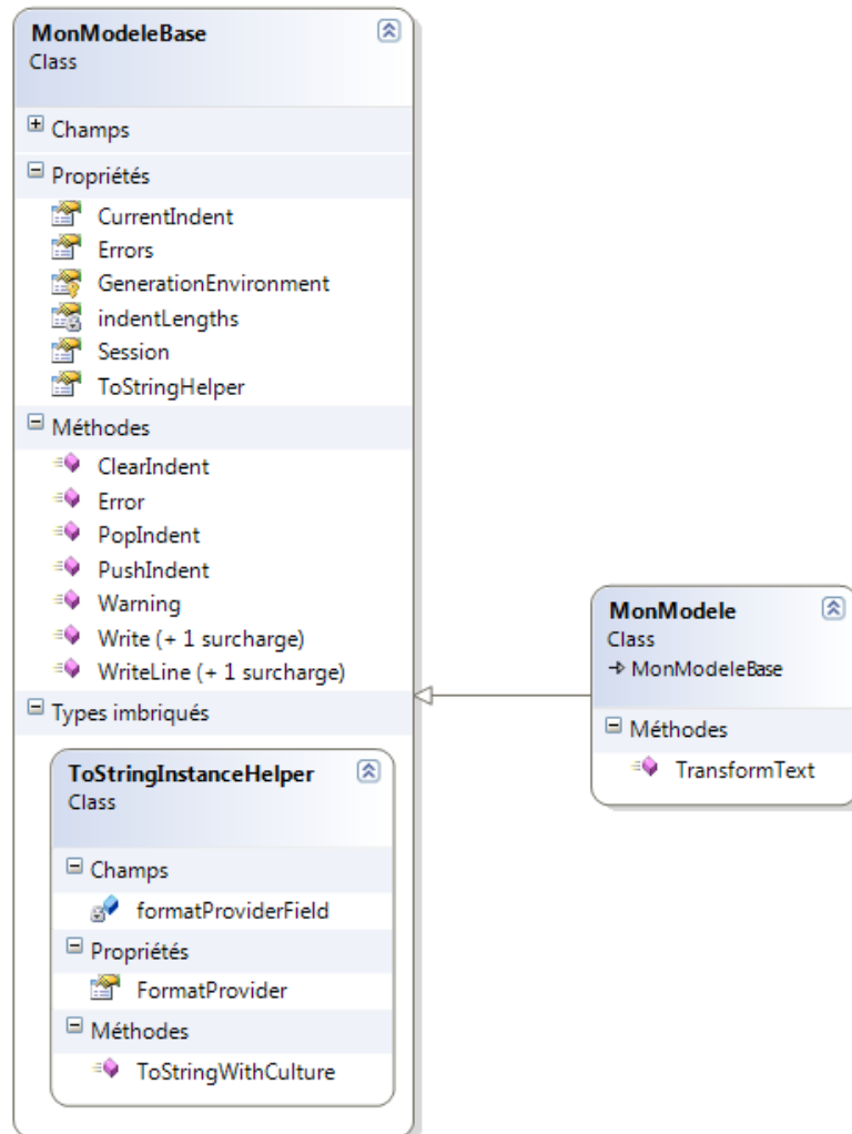
Figure 26 - Classe générée par le modèle T4 "Run Time"
