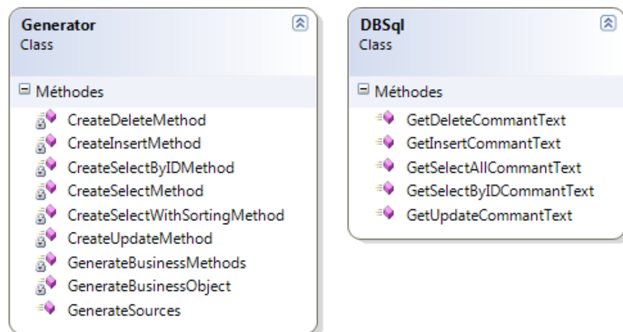
Figure 51 - Diagramme de classes - Génération du code source par la couche ORM
