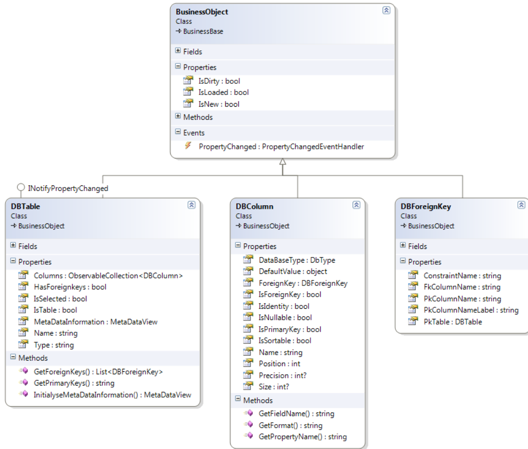
Figure 50 - Diagramme de classes représentant des métadonnées de la base de données
