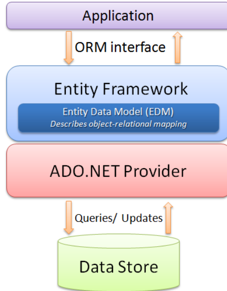
Figure 16 - Schéma d'architecture d'Entity Framework
