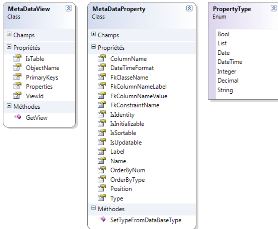
Figure 64 - Diagramme de classes - Représentation des métadonnées d'un contrôle personnalisé
