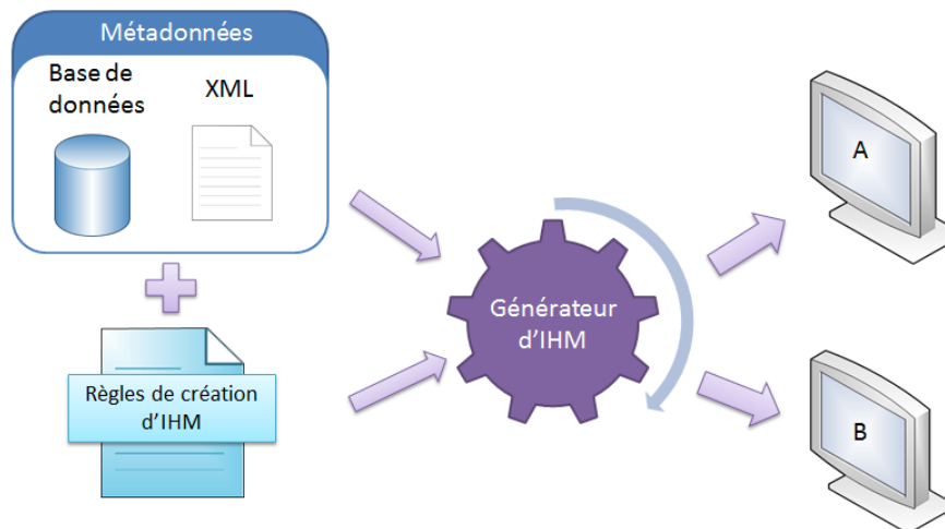
Figure 38 - Technique de génération de formulaire à l'aide de métadonnées
