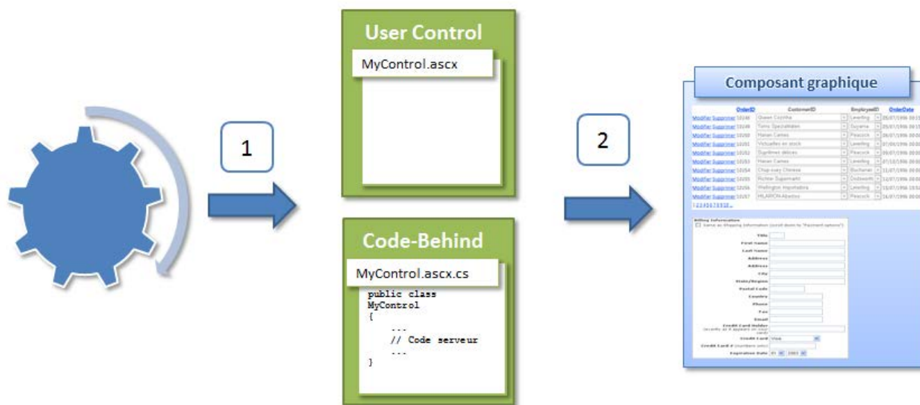
Figure 59 - Processus de génération et d'exécution du formulaire
