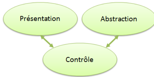
Figure 35 - Composition modèle PAC
