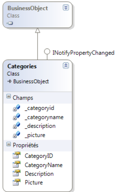
Figure 52 - Diagramme de classes - Exemple de classe "entité" générée
