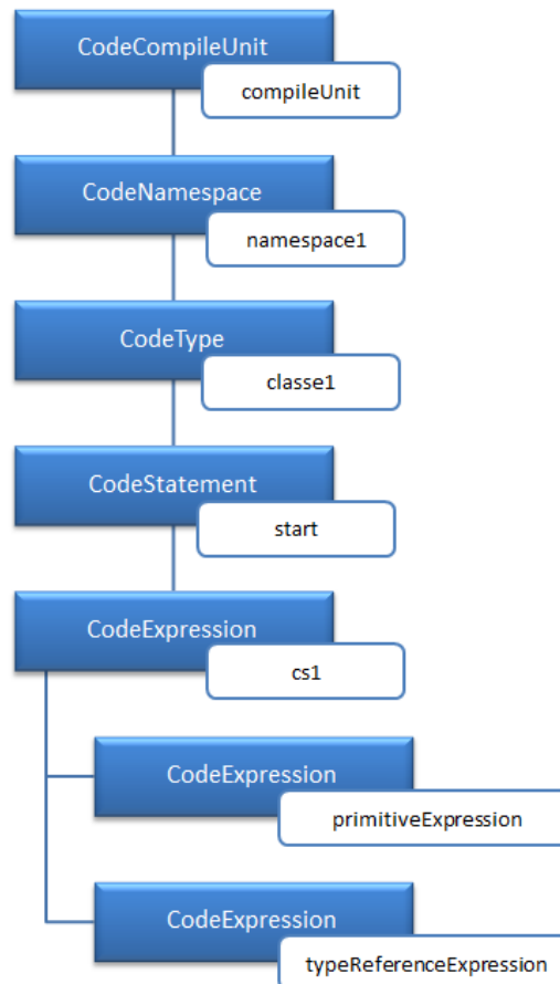
Figure 32 - Exemple d'un arbre dans CodeDOM
