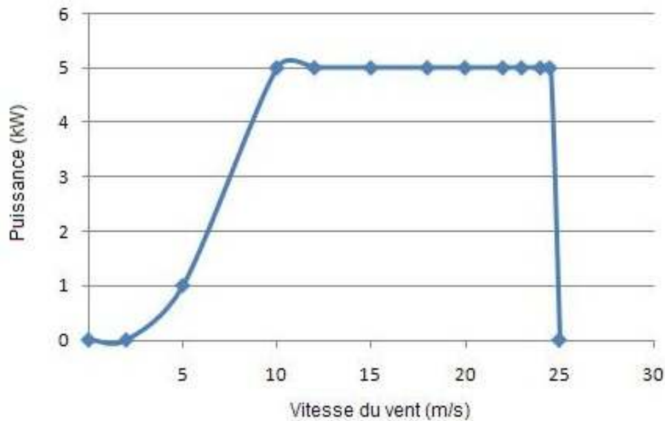
Figure 28 – Courbe de puissance de la turbine
