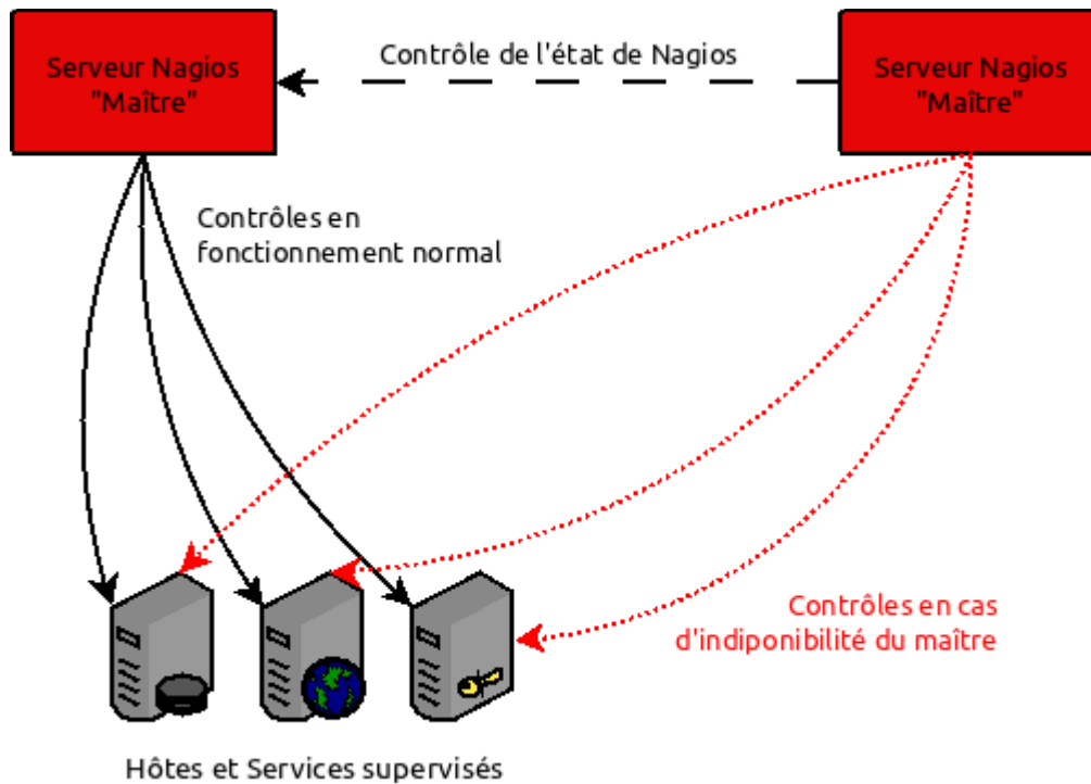
Illustration 32 : Nagios - Architecture Haute Disponibilité
