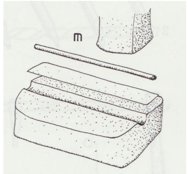
Figure 37 : Martelage d'un fil d'or
