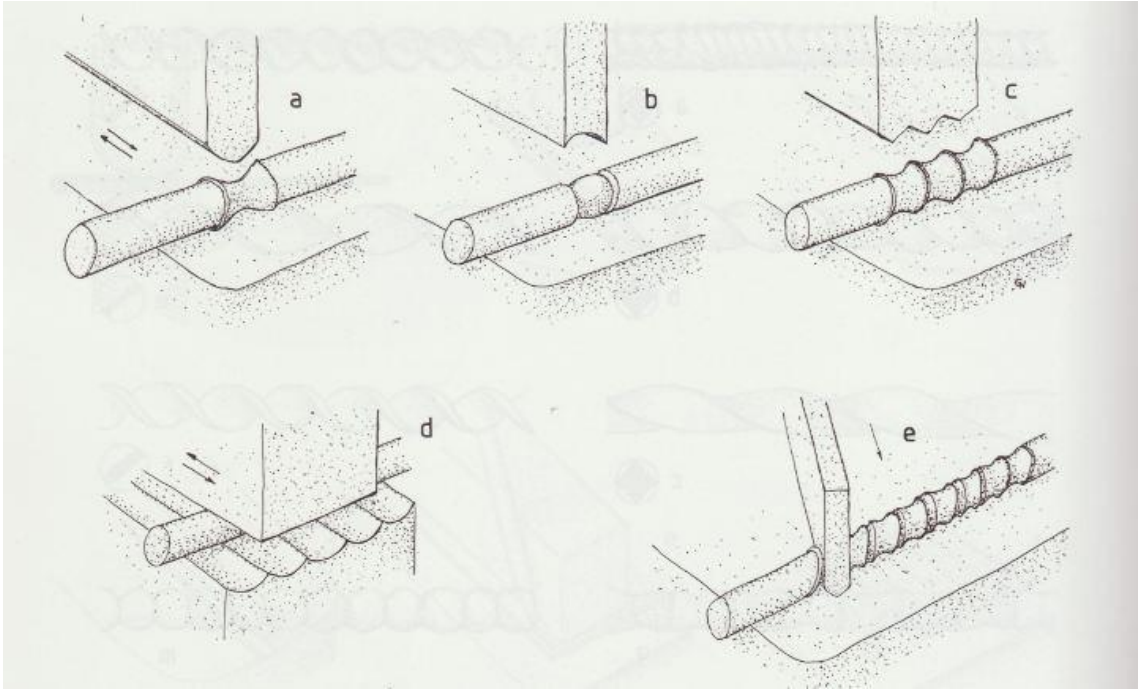
Figure 38 : Façonnage des fils
