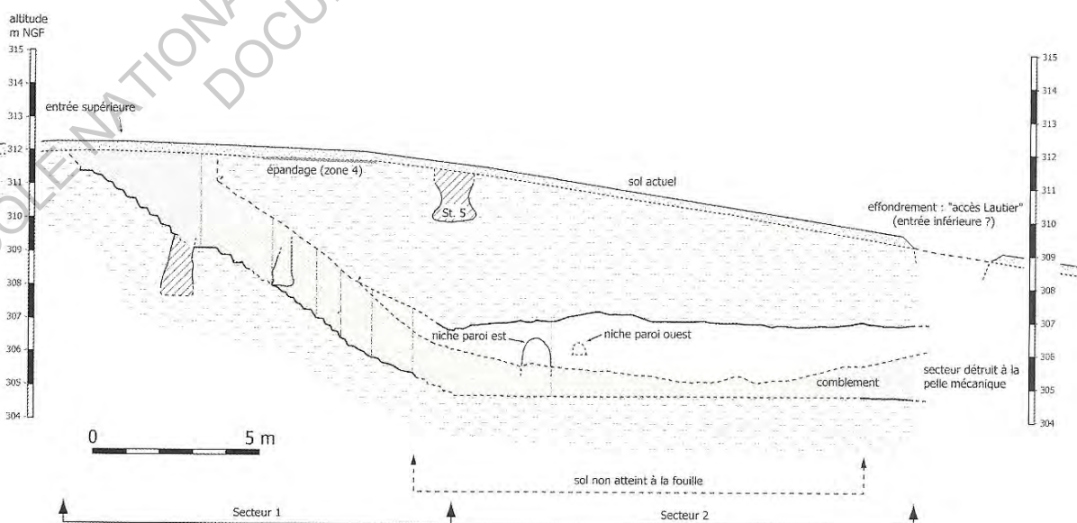
Figure 8 : Coupe du souterrain aménagé du Colombié, type Ségala (Tarn, Midi-Pyrénées)
