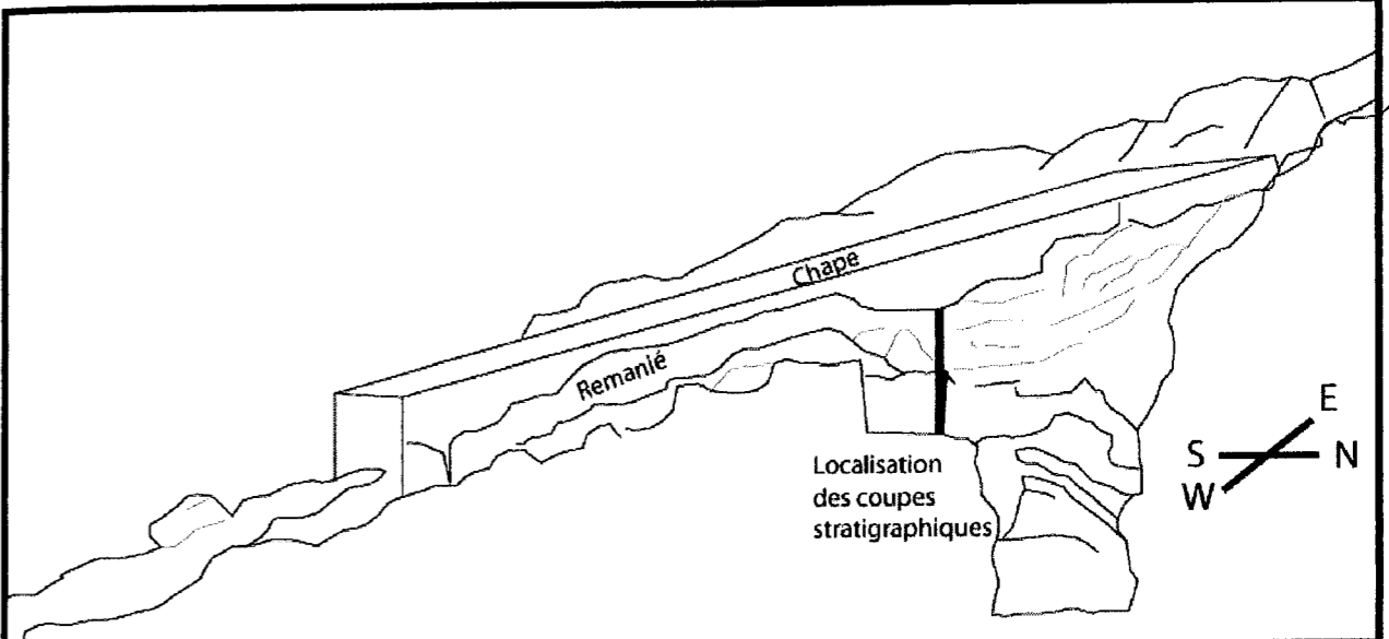
Fig.3- Vue en coupe du site de la Cueva del Angel (d'après le relevé de Daniel Botella-Ortega et al.)
