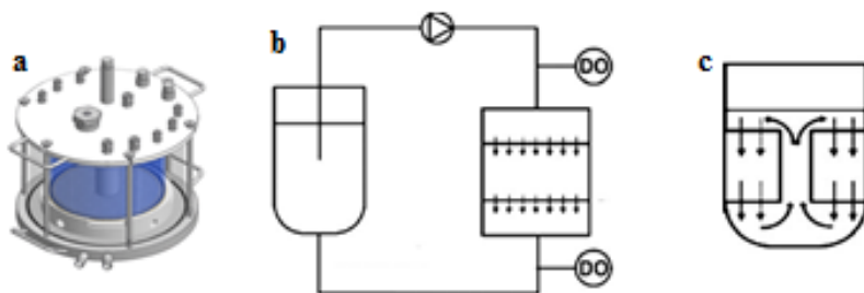
Figure 28 : a : Illustration d'un bioréacteur à lit fixe. Représentation schématique d'un bioréacteur à lit fixe : b : externe et c : interne.
