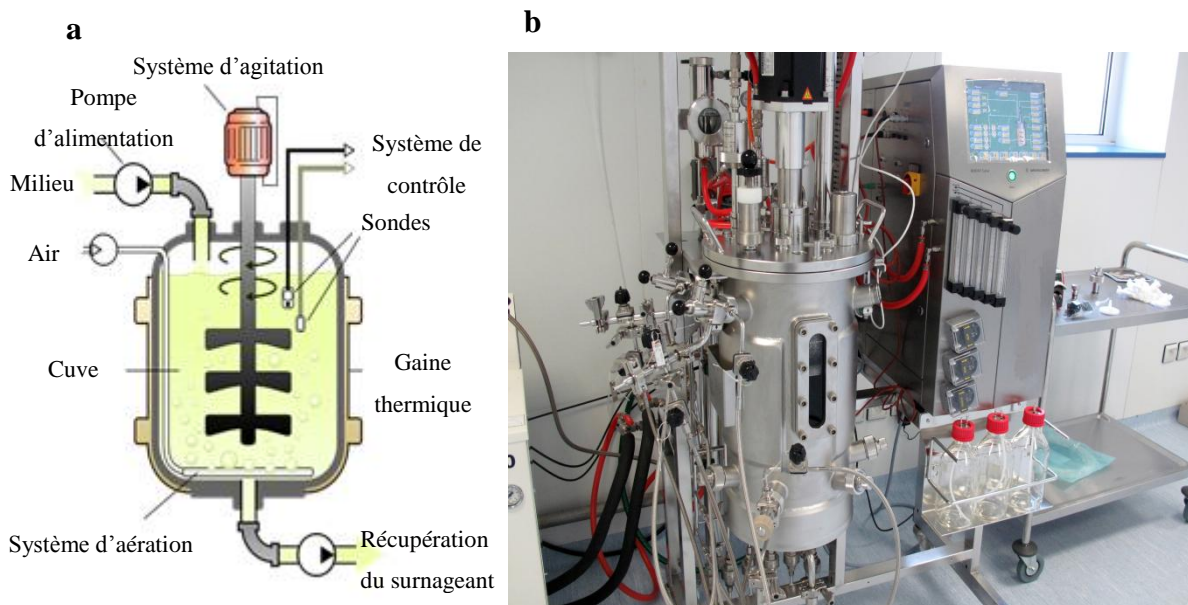
Figure 23: a : Principe d'un STR. b : Bioréacteur Inox 30 L Biostat Sartorius.
