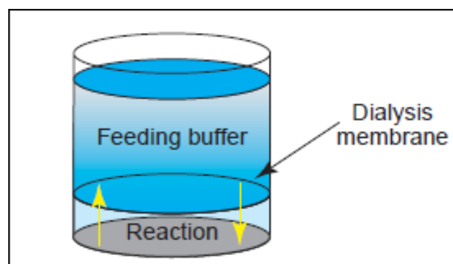
Figure 32: Schéma de la technique de Continuous Exchange Cell Free. Les flèches Jaunes indiquent le mouvement des éléments du tampon de nutrition. D'après Katzen et al 2005.
