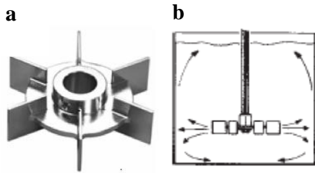
Figure 30 : a : Turbine Ruhston. b : Flux radial.
