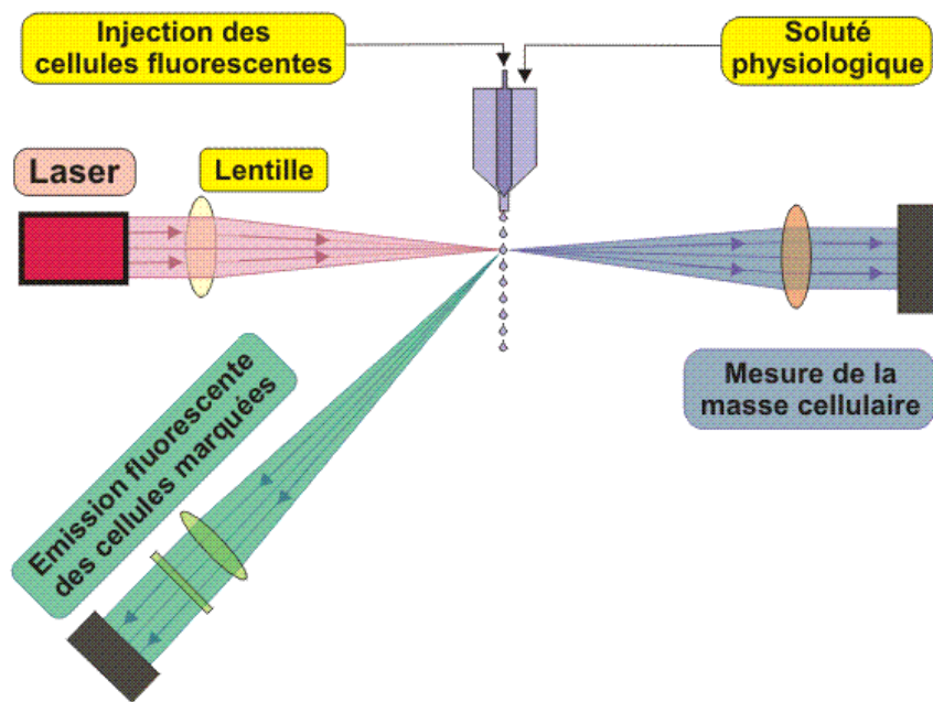
Schéma 8 : Illustration des principes de fonctionnement de la cytométrie en flux [32].
