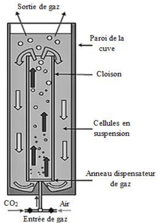
Figure 24 : Bioréacteur « air lift ».
