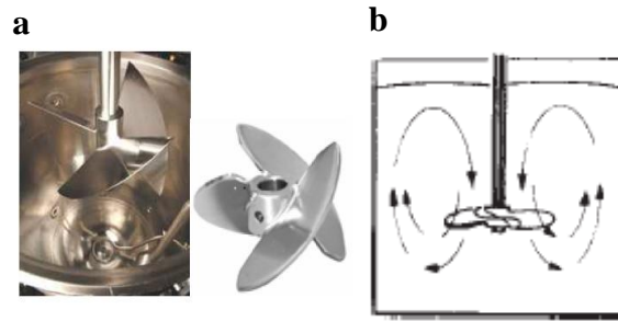
Figure 31 : a : Hélice marine. b : Flux axial.
