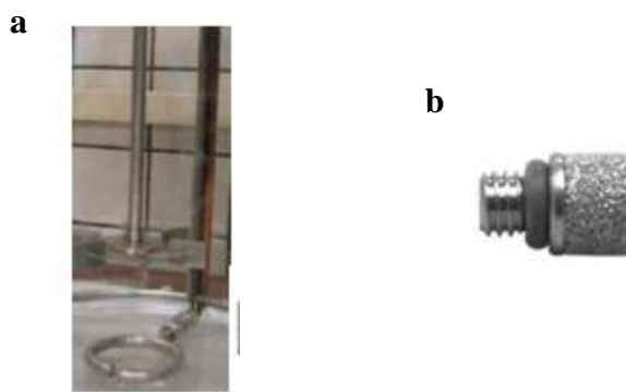
Figure 32 : a : « Ring sparger ». b : « Sparger poreux ».
