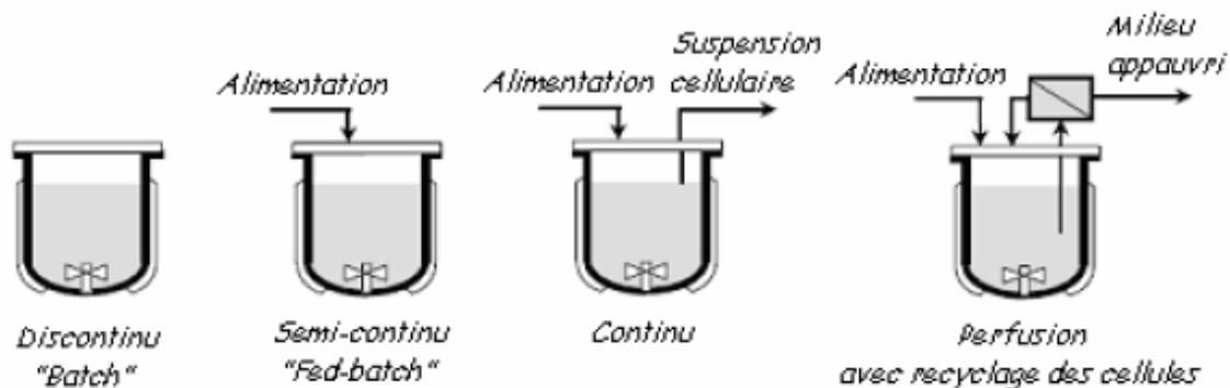
Figure 11 : Les différents modes de cultures en bioréacteurs [36].
