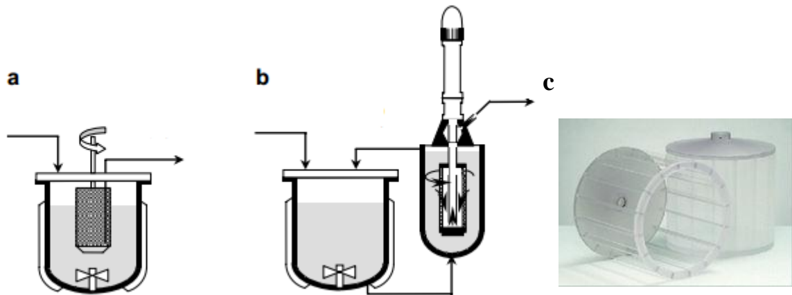
Figure 26 : Représentation schématique d'un procédé de culture par perfusion à l'aide d'un filtre rotatif. a : « spin-filter » interne ; b: « spin-filter » externe ; c : « spin-filter ».
