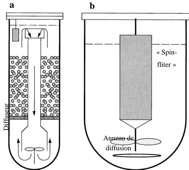
Figure 29 : Illustration schématique : a : Bioréacteur à lit fluidisé. b : STR [49].
