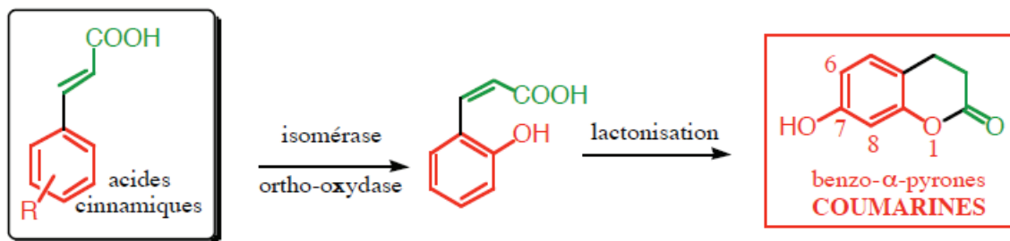
Figure 41 : Formation des coumarines par lactonisation des cinnamates (VERCAUTEREN J., 2006)
