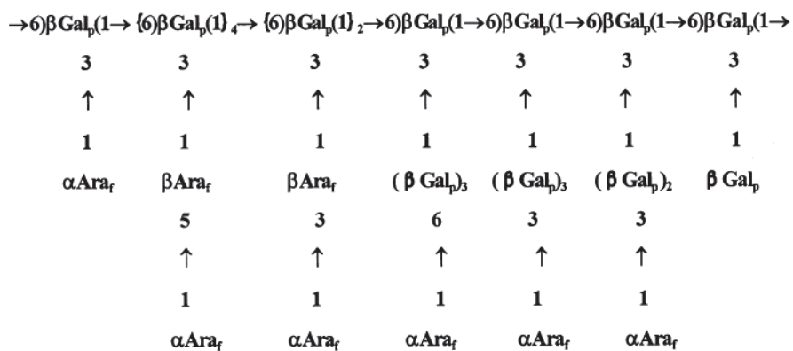
Figure 85 : Structure des polysaccharides de Lycium barbarum L. : le Lb Gp 2 (PENG X. et TIAN G., 2001)
