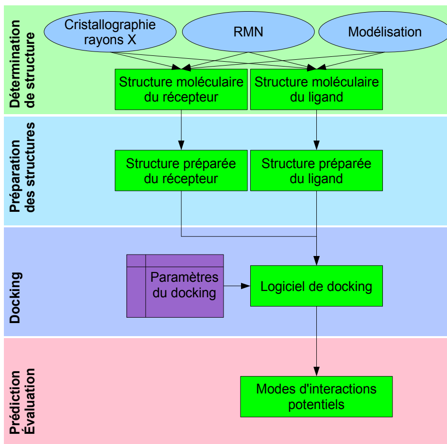
Figure 1 : Étapes typiques d'un docking. Voir détails dans le texte.
