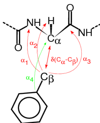
Figure 13 : Distance et angles mesurés pour évaluer la possibilité de connexion entre un backbone peptidique (en haut) et une chaîne latérale potentielle (en bas).
