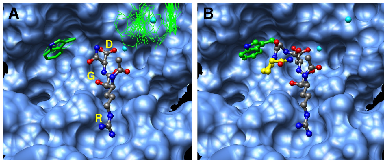
Figure 17 : (A) le peptide RGDSP (boule/bâton) positionné à la surface de l'intégrine \alpha 5\beta 1 . Les résidus S et P ne sont pas montrés par souci de clarté de la figure. Les positions favorables de la chaîne latérale du tryptophane sont visibles sous forme de fine ligne verte, excepté le plus favorable en représentation bâtonnets verts. (B) Mode d'interaction calculé par EADock pour le peptide linéaire RGDWP.
