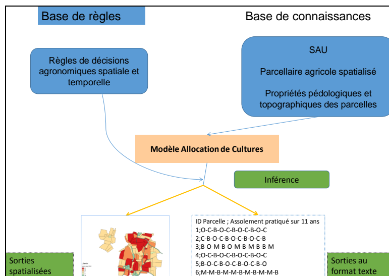
Figure 3: Fonctionnement du modèle décisionnel
