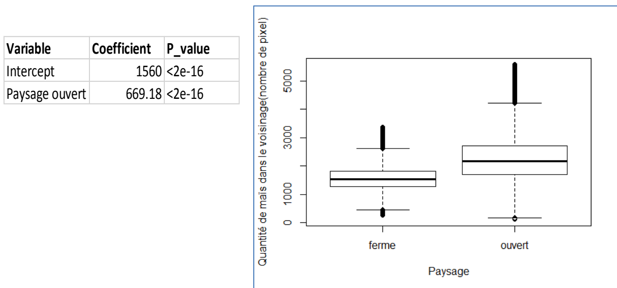
Figure 17 : Effet du paysage sur la variabilité de la métrique
