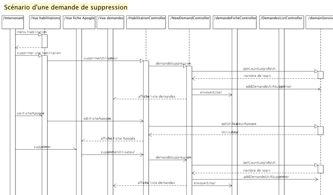
Figure 68 Diagramme de séquence d'une demande de suppression Source : MC COLLAS
