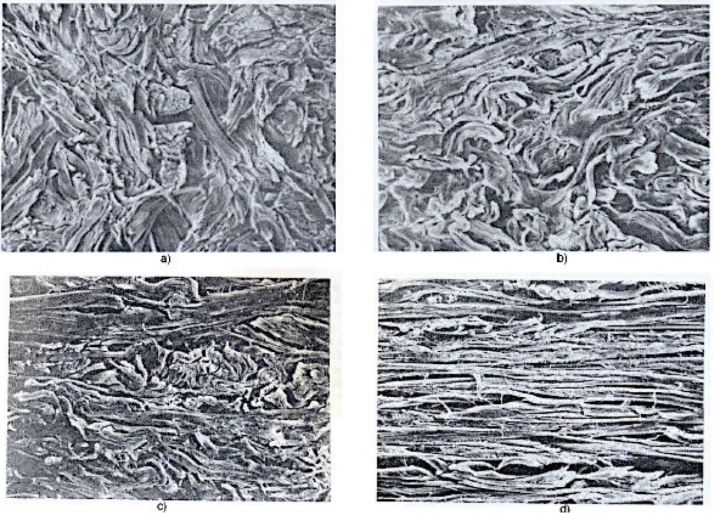
Figure 16 : Fibres de collagène en traction uni axiale : a) Etat initial, b) Phase 1, c) Phase 2, d) Phase 3.
