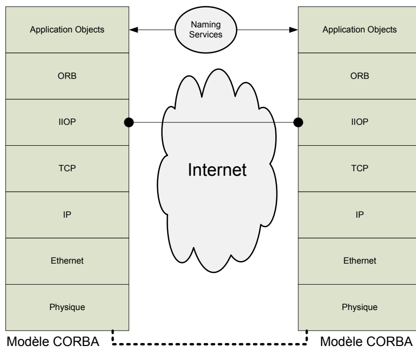
Figure 18 : couches de communication du modèle CORBA
