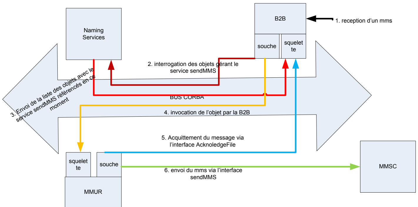
Figure 19 : Echange entre deux machines
