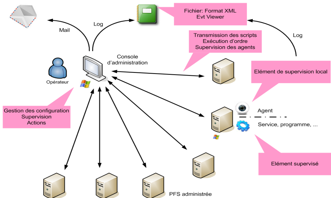
Figure 8 : Dialogue avec ISC
