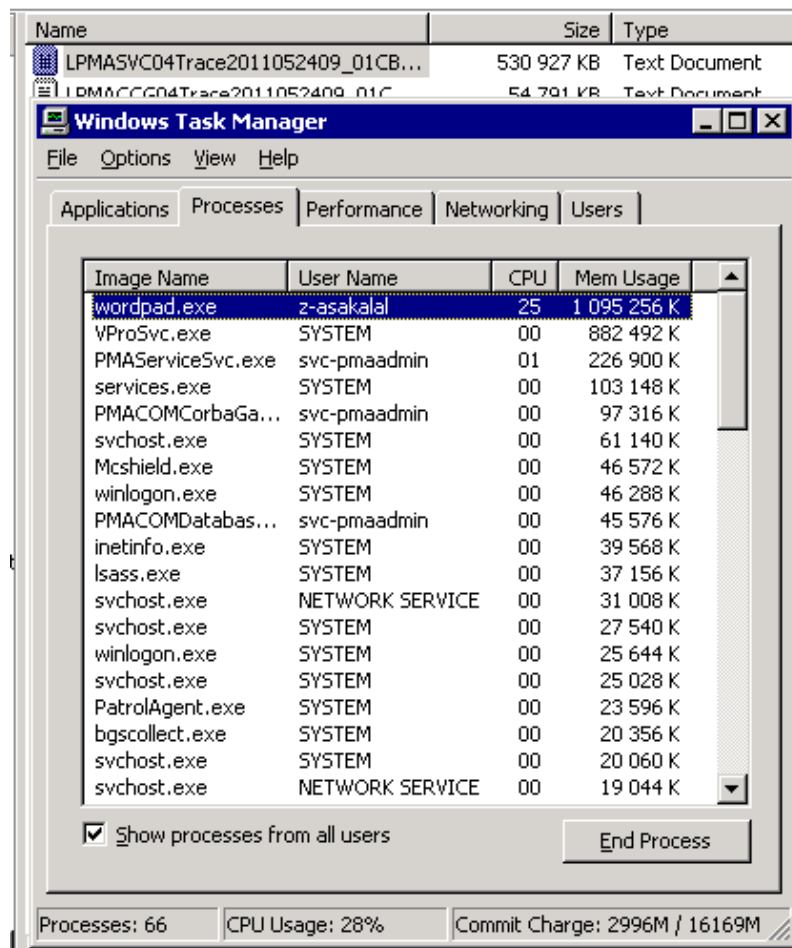
Figure 22 : Gestionnaire de tâches PMA(2)
