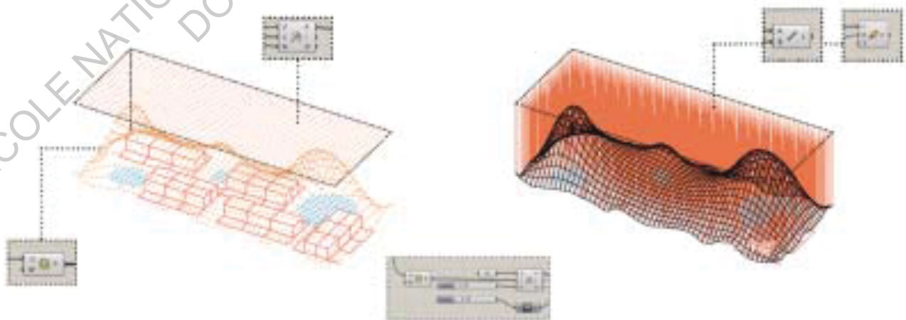
Schéma explicatif de la génération formelle – Création du nuage cinétique Liaison de la trame inférieur et supérieure par des tiges verticales / Grasshopper
