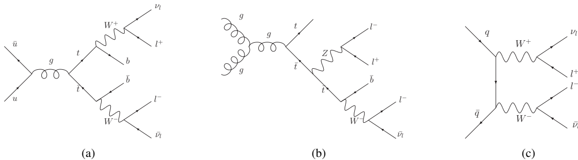
FIG. 4.1: Bruits de fond t\bar{t} (a), t\bar{t}V (b) et Dibosons (c).
