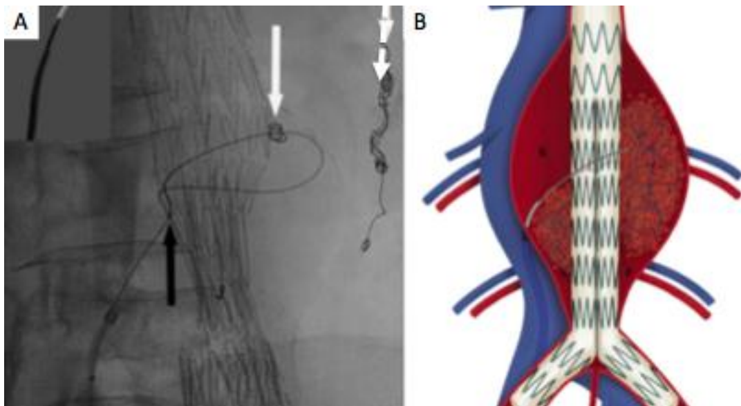
Figure 19- Embolisation trans-cave (156).
