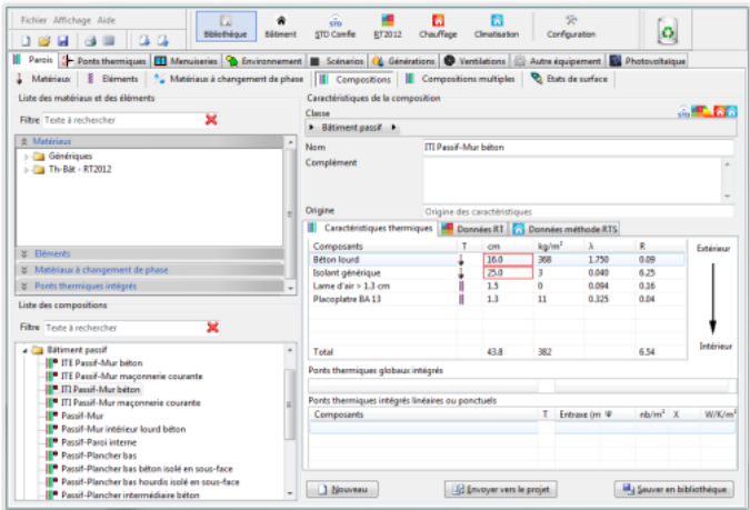
Figure 9 : Fenêtre de création d'une paroi dans PLEIADES
