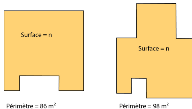
Figure 27 : Différence de surface déperditive pour un même volume mais pour des formes de bâtiments différentes. Vues en plan
