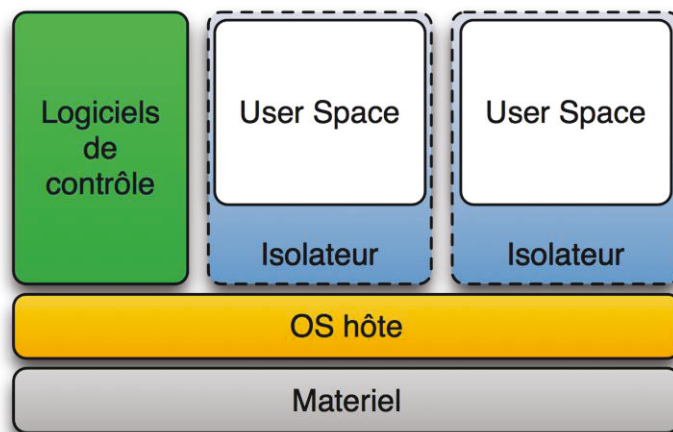
Figure 8 – Isolateur (Source : Wikipédia)
