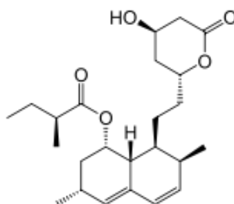
Figure 14 : Structure d'un polycétide d'intérêt thérapeutique : la lovastatine
