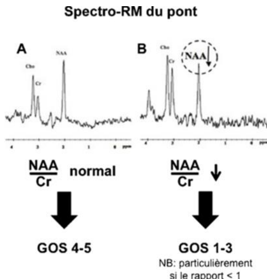
Figure 6 : Spectroscopie par résonance magnétique du pont
