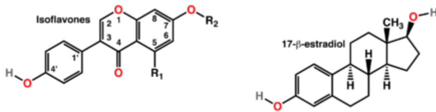
Figure 26 : Comparaison des structures du 17- \beta œstradiol et des isoflavones [57]
