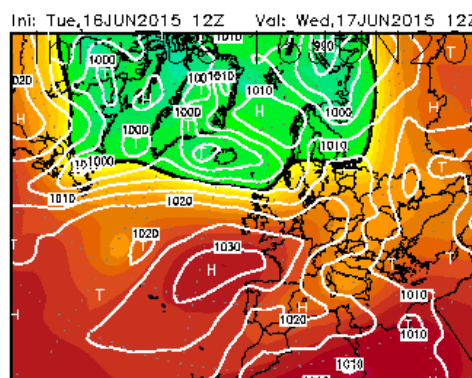
Figure 9. Carte de prévision météorologique basée sur le Z500. Adaptée de : http://www.wetterzentrale.de .
