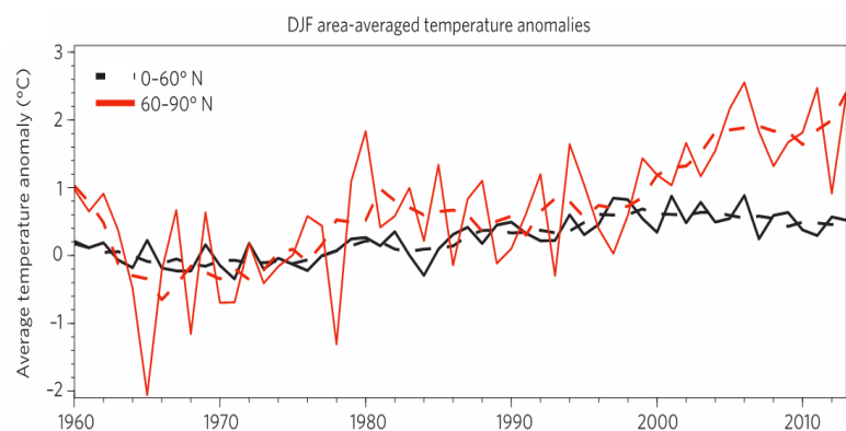
Figure 5. Moyenne des anomalies de température de surface ( ^\circ C ) entre 0 - 60^\circ N (en noir) et 60-90^\circ N (en rouge) avec un lissage sur 5 ans (respectivement en noir et rouge pointillé). Une anomalie de température d'environ +2^\circ C est observable au niveau des hautes latitudes à partir de la fin des années 1990. Source : Cohen et al. , 2014.
