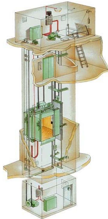
Fig.5: Vue générale des composants d'un ascenseur
