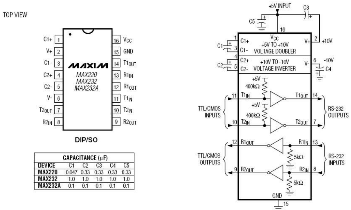
Fig.30: Le MAX232
