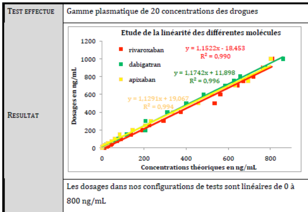
Figure 39 : Etude de linéarité des méthodes de dosage « maison » des différents AODs, (Thèse de D. Girard, juin 2015) (59)
