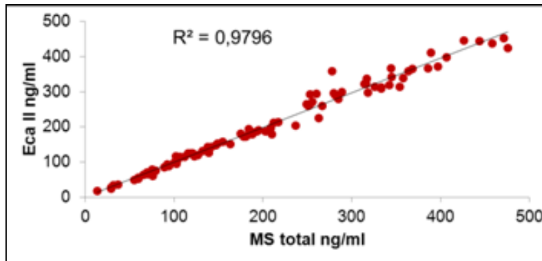
Figure 32 : Corrélation entre le dosage du dabigatran réalisé par ECAII et HPLC-MS/MS au CHU de Bordeaux, (G. Freyburger 2015) (66)
