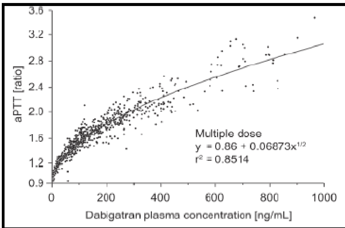
Figure 29 : Evolution du TCA en fonction de la concentration en dabigatran (J. van Ryn, 2010) (63)
