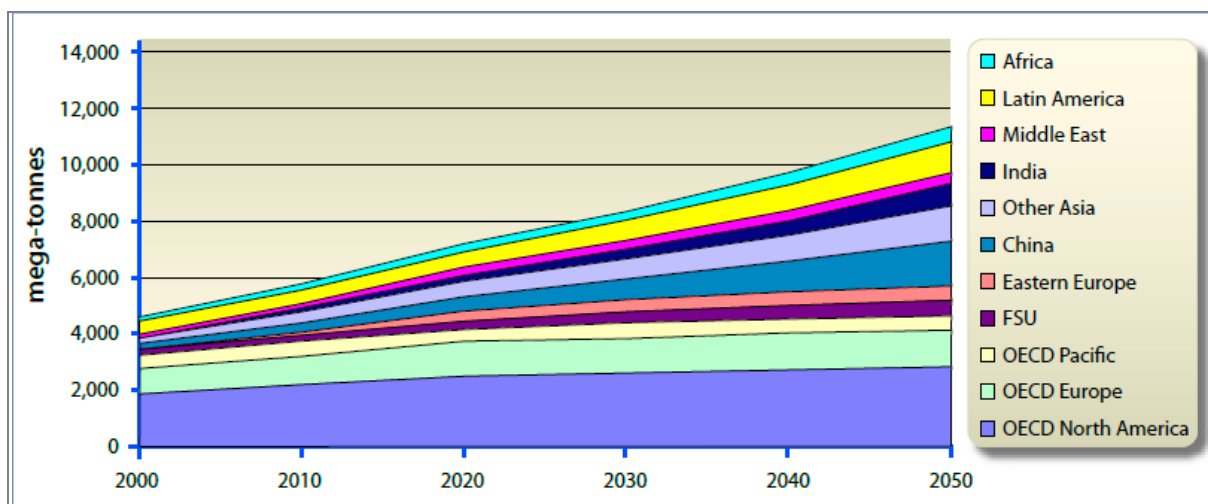
Figure 9 : Tendances pour différentes régions du monde des émissions de CO 2 issues du secteur des transports (Source : Holger Dalkman, Charlotte Branningan et al., 2007)
