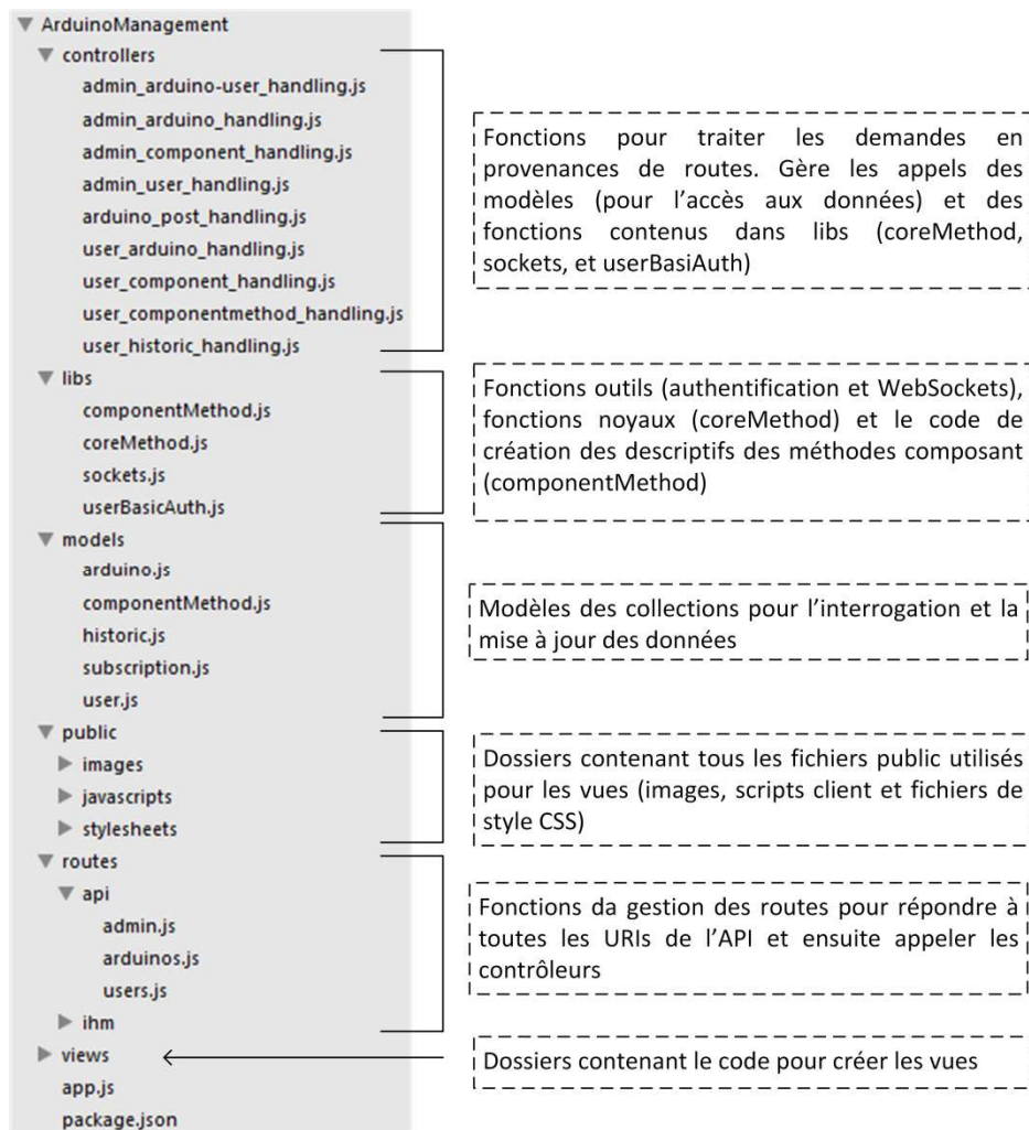
Figure 44 - Organisation du code de l'applicatif
