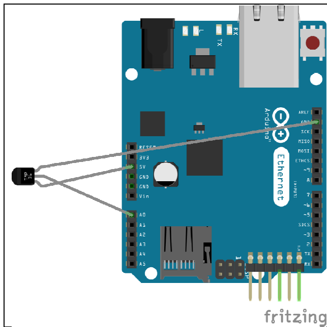
Capteur de température (TMP36)
