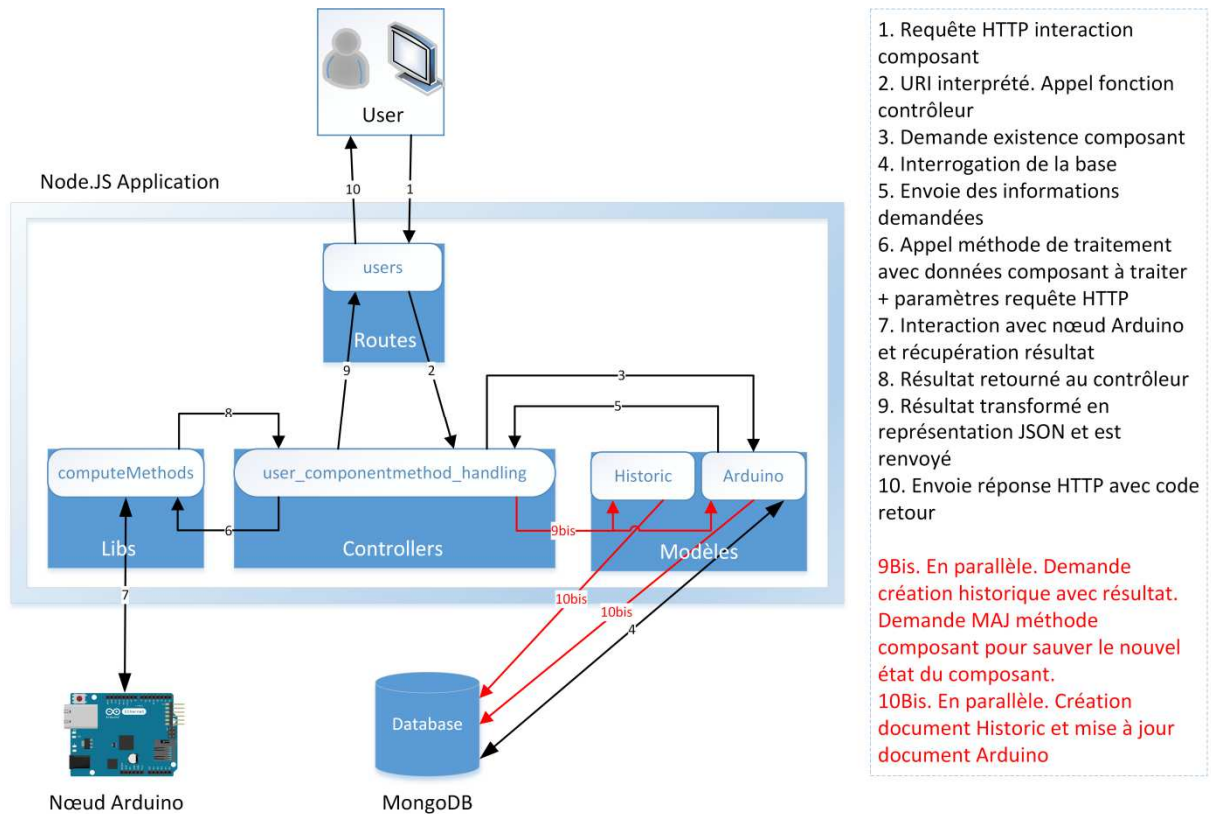
Figure 49 - Schéma d'architecture logicielle pour le fonctionnement standard
