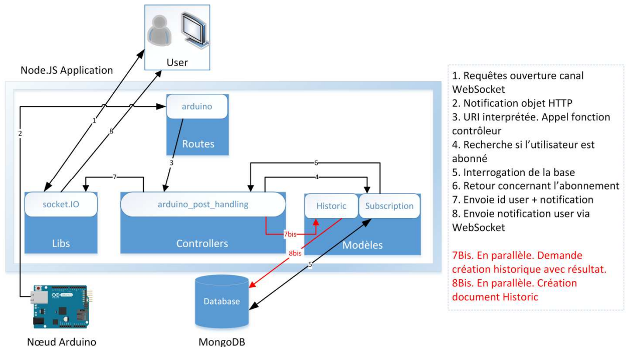
Figure 50 - Schéma d'architecture logicielle pour le fonctionnement avec événements
