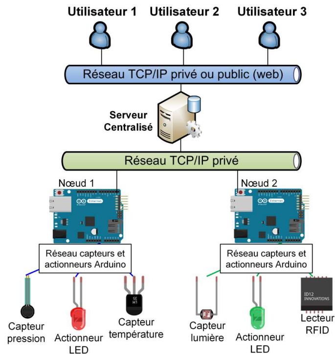
Figure 7 - Communication du système
