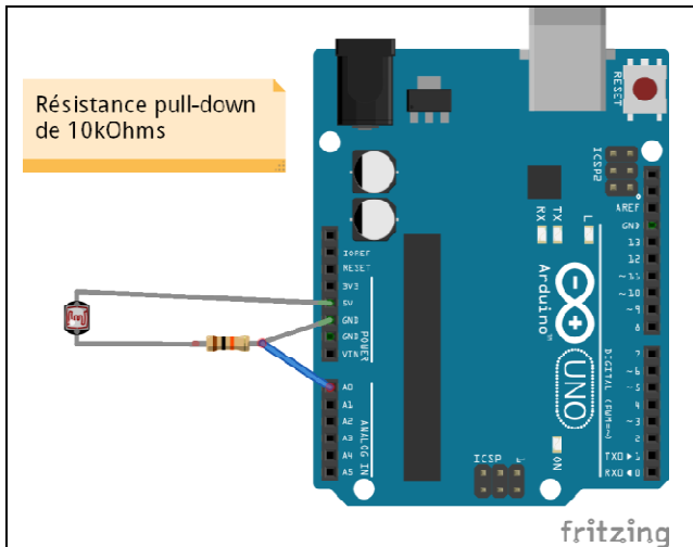
Capteur de luminosité (photoresistance)
