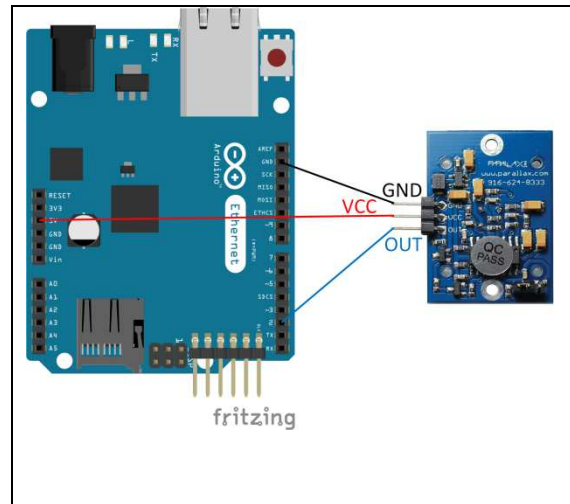
Détecteur de mouvement (Parallax PIR Rev B)
