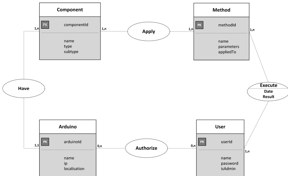
Figure 12 - Modèle entité-relation
