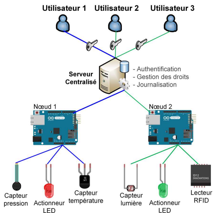
Figure 6 - Multi-utilisateurs
