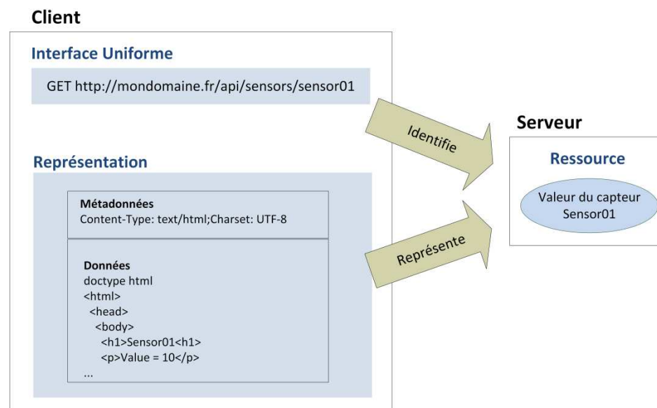
Figure 10 - Représentation REST
