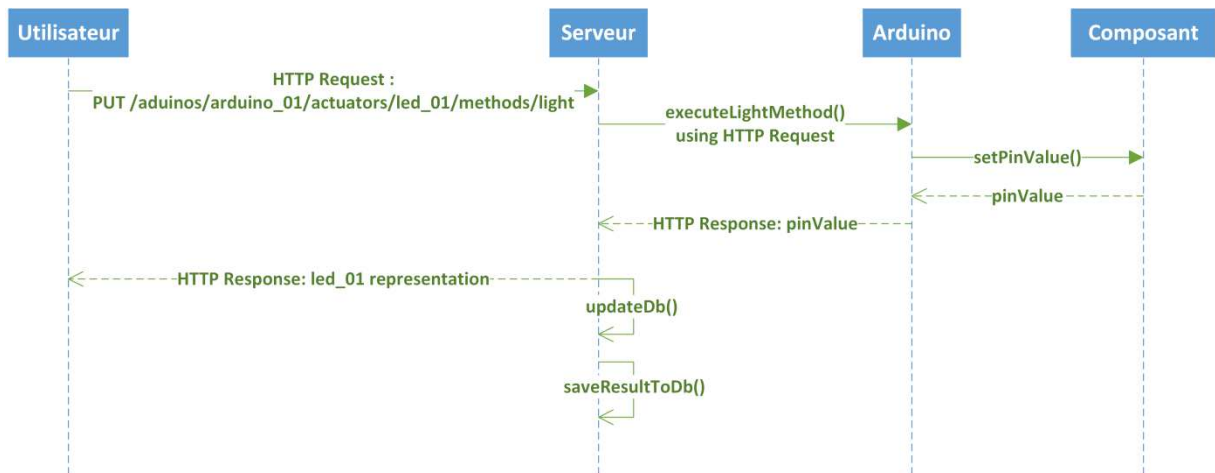
Figure 25 - Diagramme de séquence : communication unidirectionnelle
