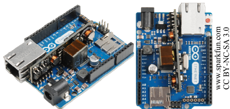
Figure 28 - Arduino Ethernet avec PoE
