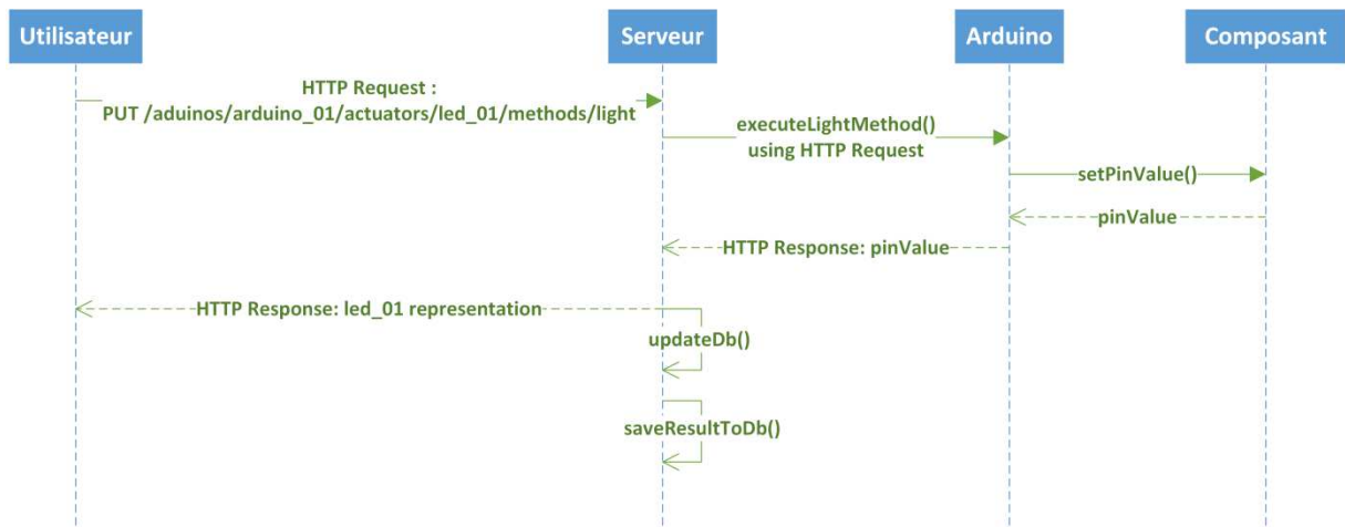
Figure 25 - Diagramme de séquence : communication unidirectionnelle
