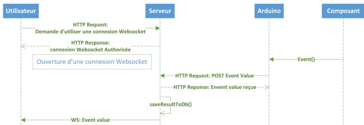
Figure 26 - Digramme de séquence : communication bidirectionnelle
