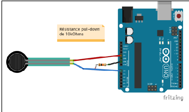
Capteur de pression
