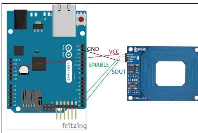
Lecteur RFID (Parallax 28140)
