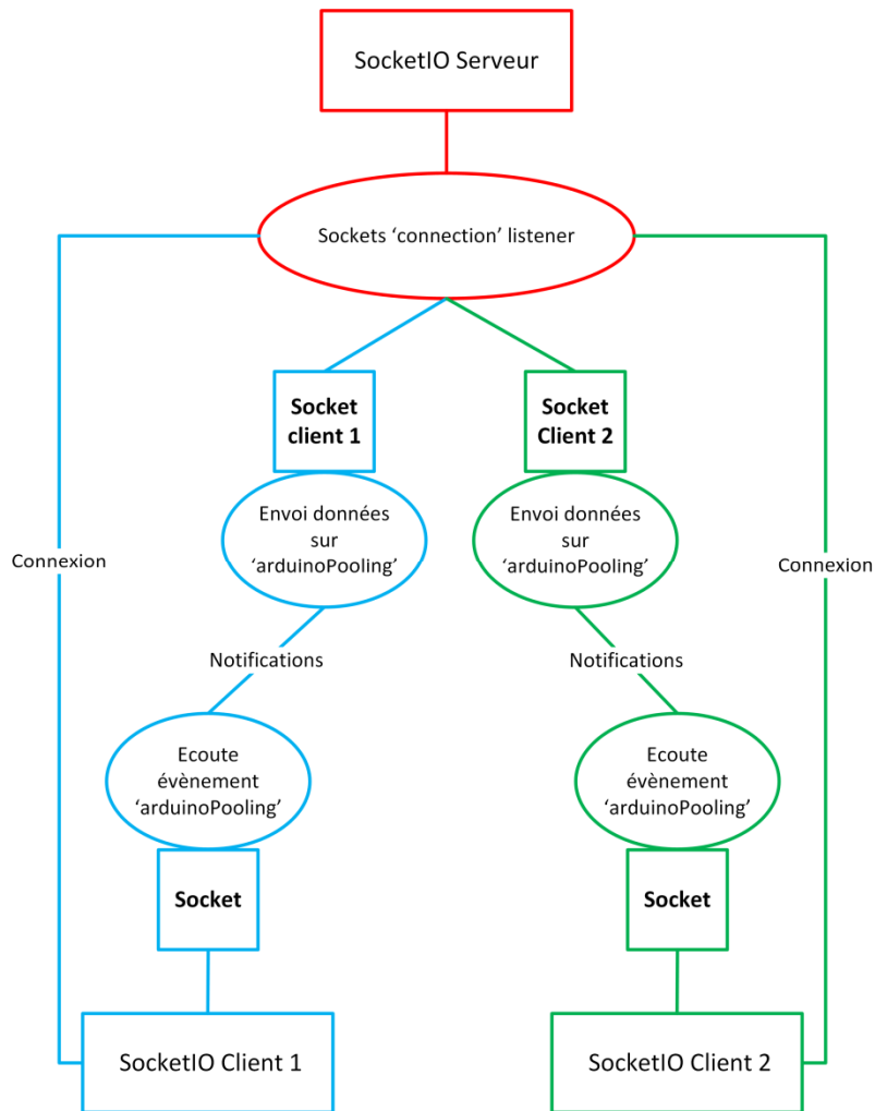
Figure 48 - Fonctionnement Socket.IO pour les notifications Arduino
