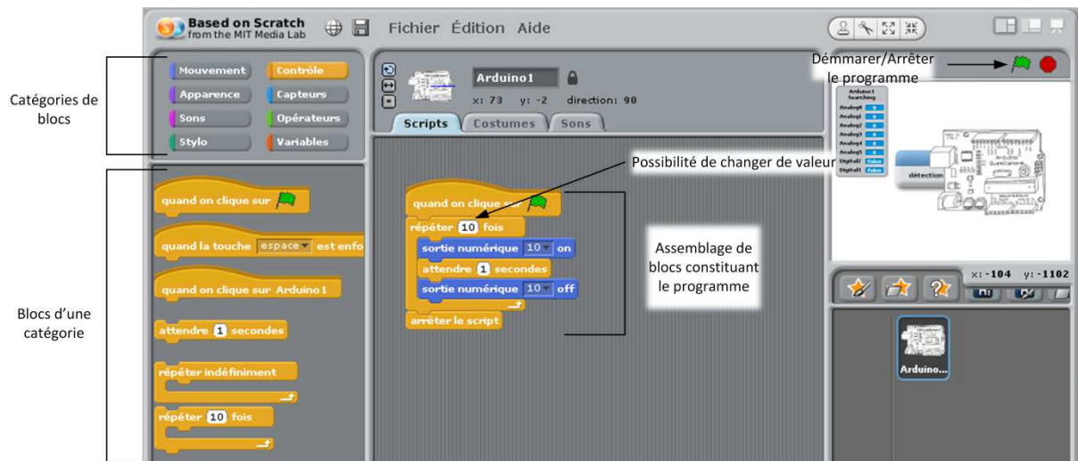
Figure 61 - Programmation visuelle avec S4A
