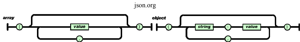
Figure 39 - Objet et tableau JSON
