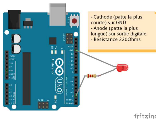
Figure 51 - Schéma Fritzing pour LED
