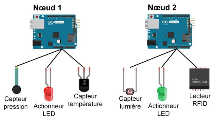
Figure 4 - Nœud de capteurs et d'actionneurs
