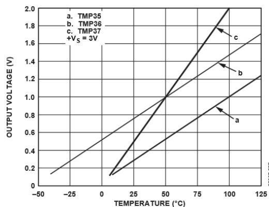
Figure 38 - TMP36 : voltage en fonction de la température [TMP36 Data Sheet – 2015]
