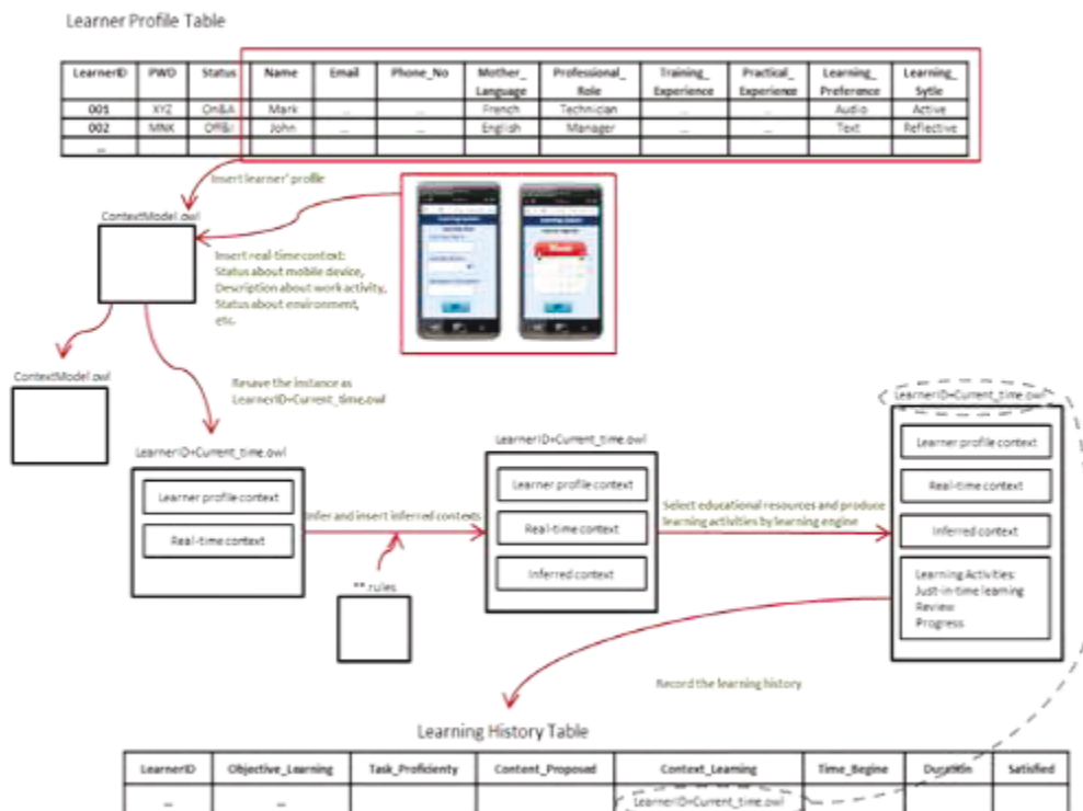
FIGURE 19 : PROCESSUS DE PRODUCTION DU FICHIER DE CONTEXTE D'APPRENTISSAGE
