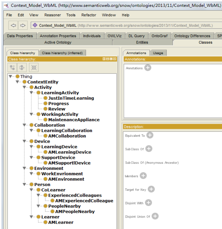
FIGURE 14 : CONSTRUIRE UNE CLASSE AVEC PROTEGE
