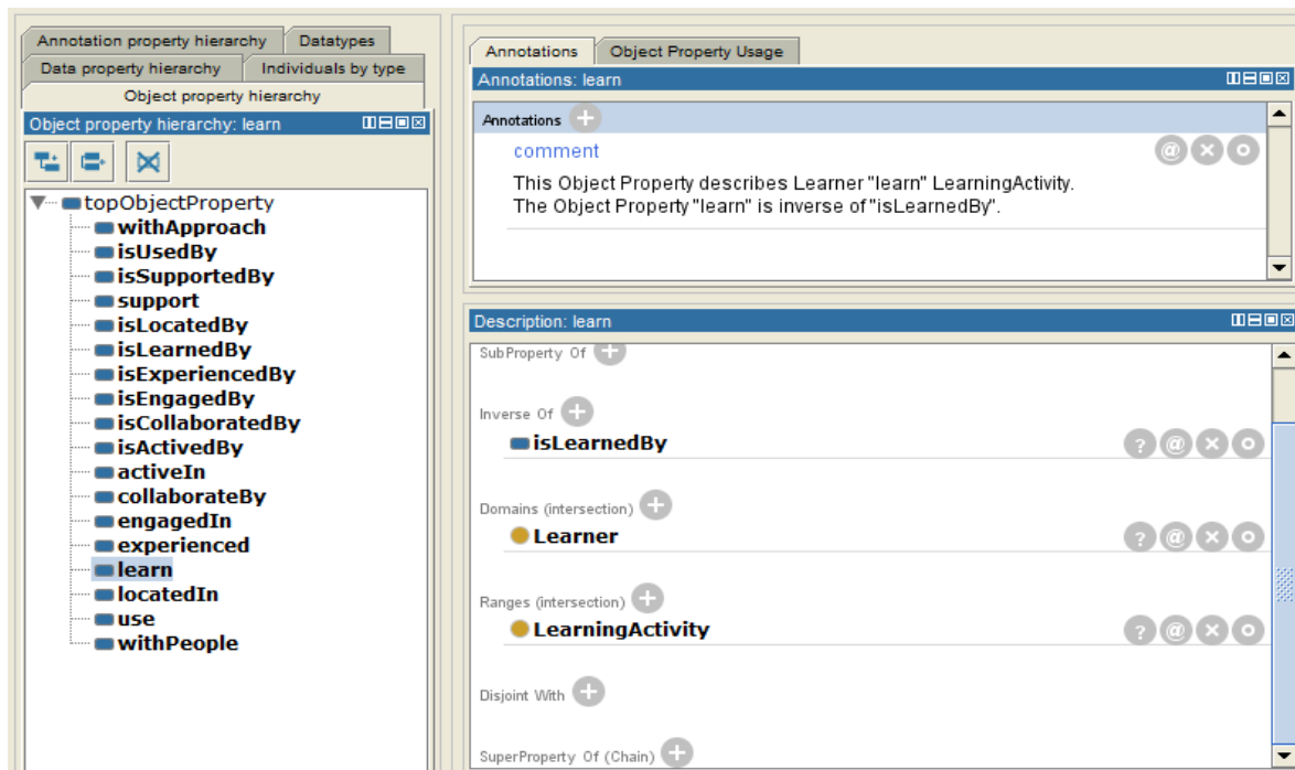
FIGURE 16 : SET OBJECTPROPERTIES AVEC PROTEGE
