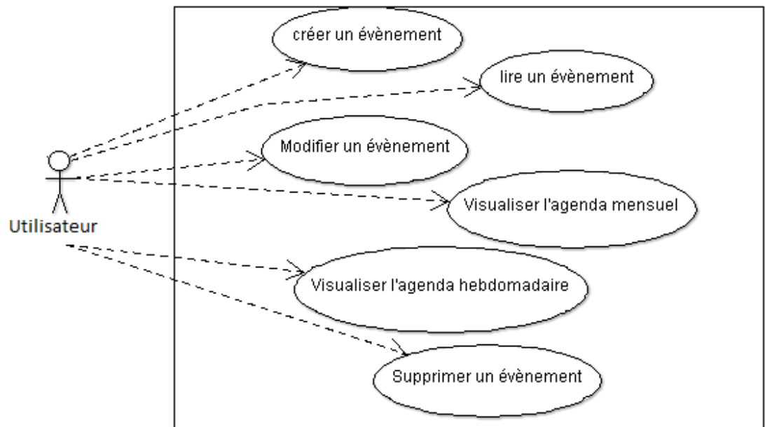
FIGURE 5 : DIAGRAMME DE CAS D'UTILISATION AGENDA
