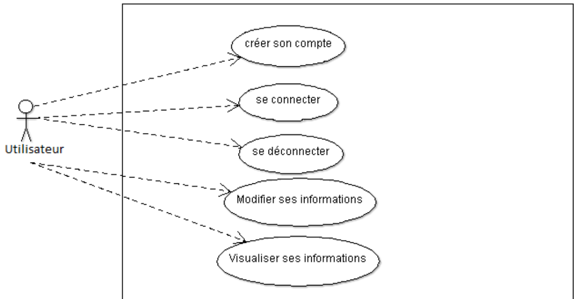
FIGURE 4 : DIAGRAMME DE CAS D'UTILISATION DE L'UTILISATEUR
