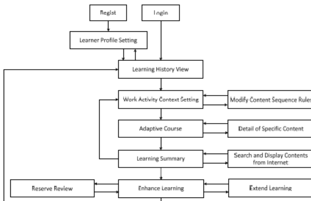
FIGURE 13 : L'ENCHAÎNEMENT D'INTERFACES HOMME-MACHINE DE NOTRE OUTIL
