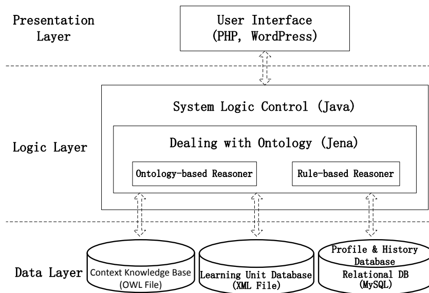
FIGURE 17: L'ARCHITECTURE FONCTIONNELLE DU WOBALearn
