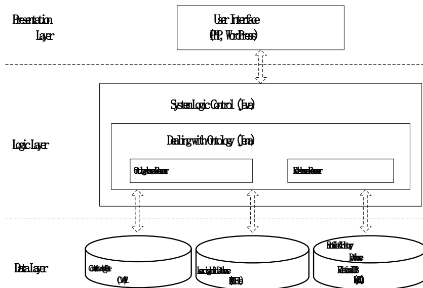
FIGURE 12 : L'ARCHITECTURE FONCTIONNELLE DU WOBALearn
