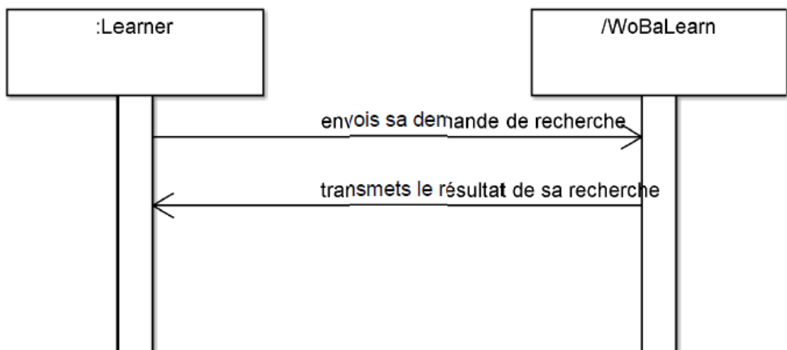
FIGURE 8 : DIAGRAMME DE SEQUENCE DU CAS DE RECHERCHE D'UNE FORMATION
