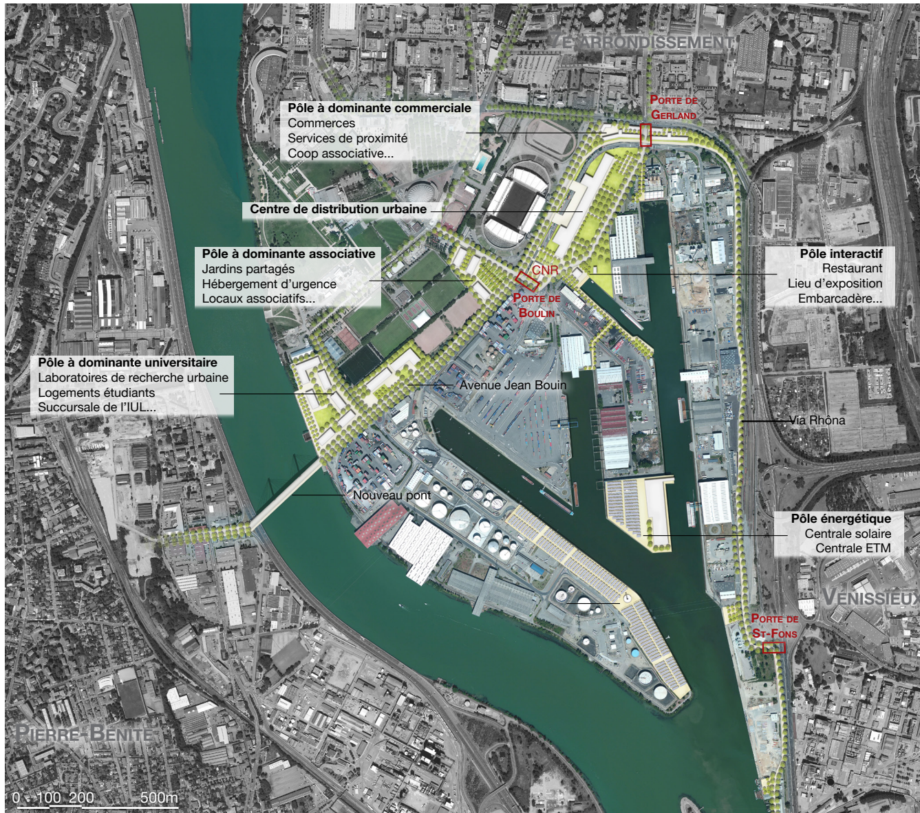
Plan masse du port Edouard Herriot
