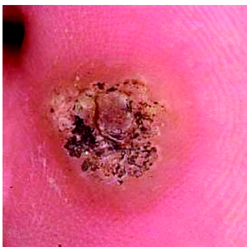
Figure 7 : Myrmécie
