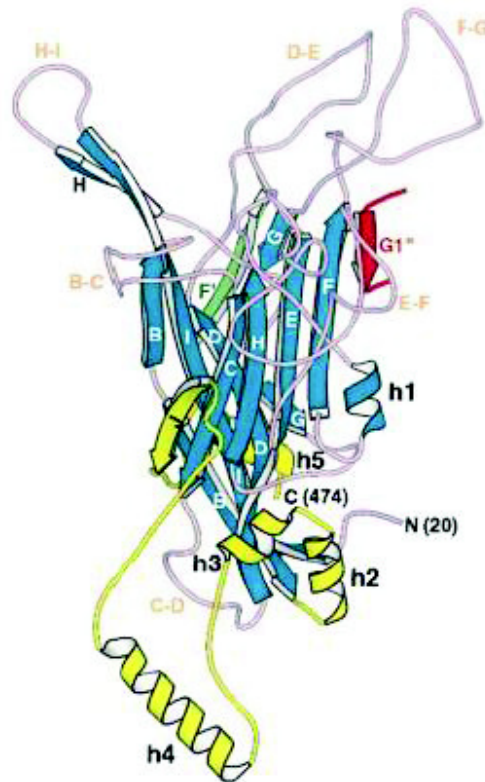
Figure 21 : Protéine L1
