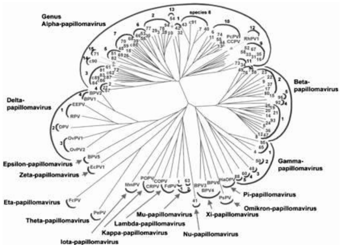
Figure 1 : Arbre phylogénétique
