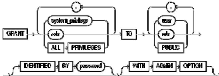
Figure 0.1 : Procédure d'assignation des privilèges système
