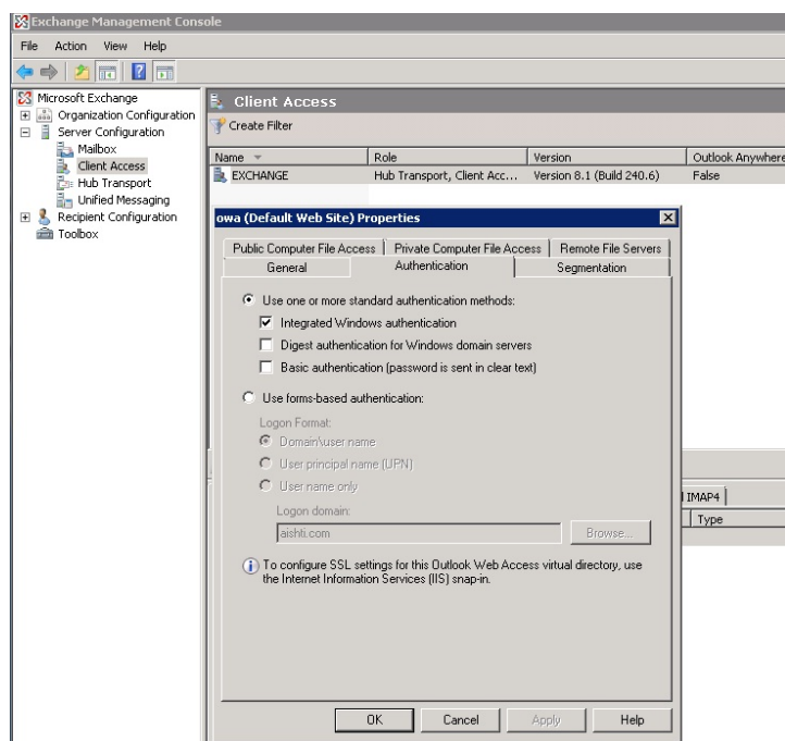
Figure 0.33 : Méthode d'authentification avec le serveur de messagerie
