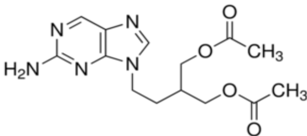
Figure 42 : Structure du famciclovir (47)
