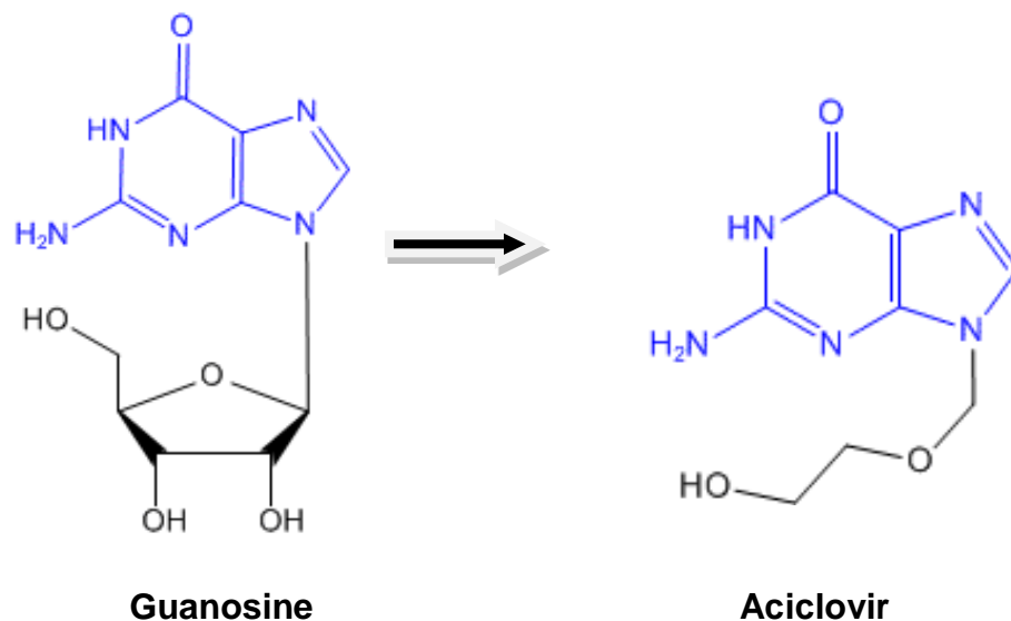
Figure 39 : Différence structurale entre guanosine et aciclovir (57)
