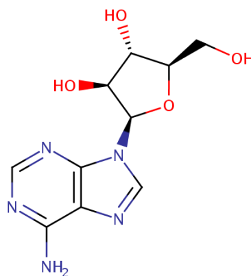
Figure 43 : structure de la vidarabine (47)
