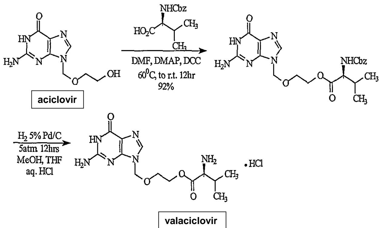
Figure 41 : Réaction d'estérification avec formation du valaciclovir (57) 9-(2-hydroxyéthoxyméthyl) guanine estérifiée par la L-valine.
