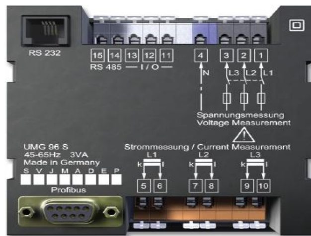
Figure III-5 : illustration de la connexion de l'appareil GANITZA UMG 96 S
