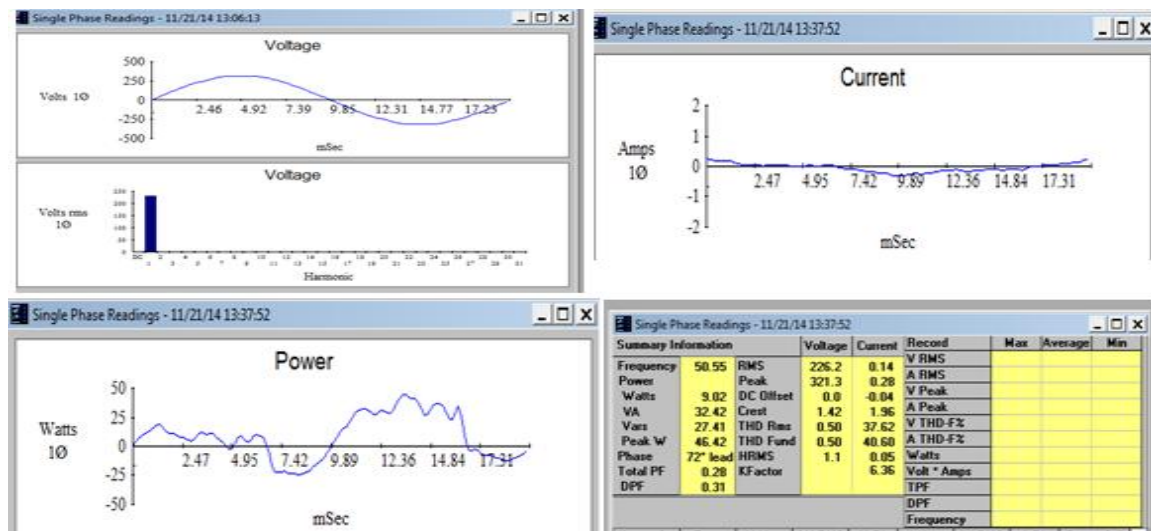
Figure B-41 : Les signaux de phase 1 des climatiseurs de deuxième étage.
