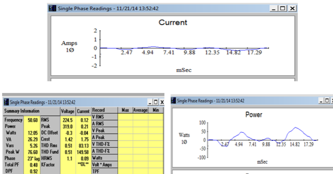
Figure B-48: Les signaux de fil neutre des climatiseurs de troisième étage.
