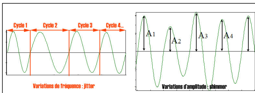
Fig. 64 : Variations instantanées des caractéristiques de la vibration à gauche, l'écart de fréquence entre deux cycles consécutifs entraînera un jitter important ; à droite, l'écart d'amplitude entre deux cycles consécutifs entraînera un shimmer important [28]
