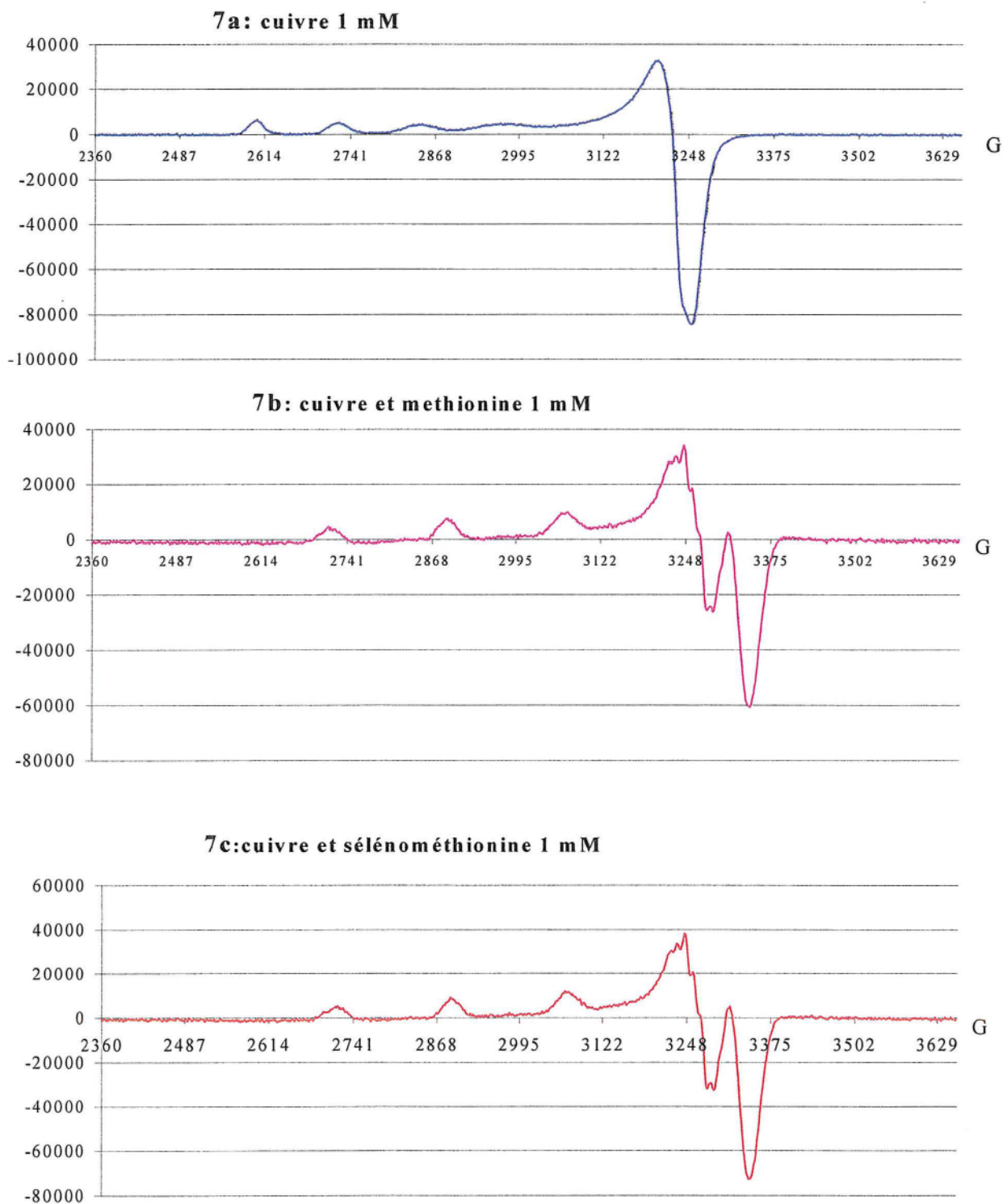
Figure n°7 : spectre RPE des acides aminés et du cuivre (a) , méthionine (b), sélénométhionine (c), cystine (d), sélénocystine (e), cystéine (f).
