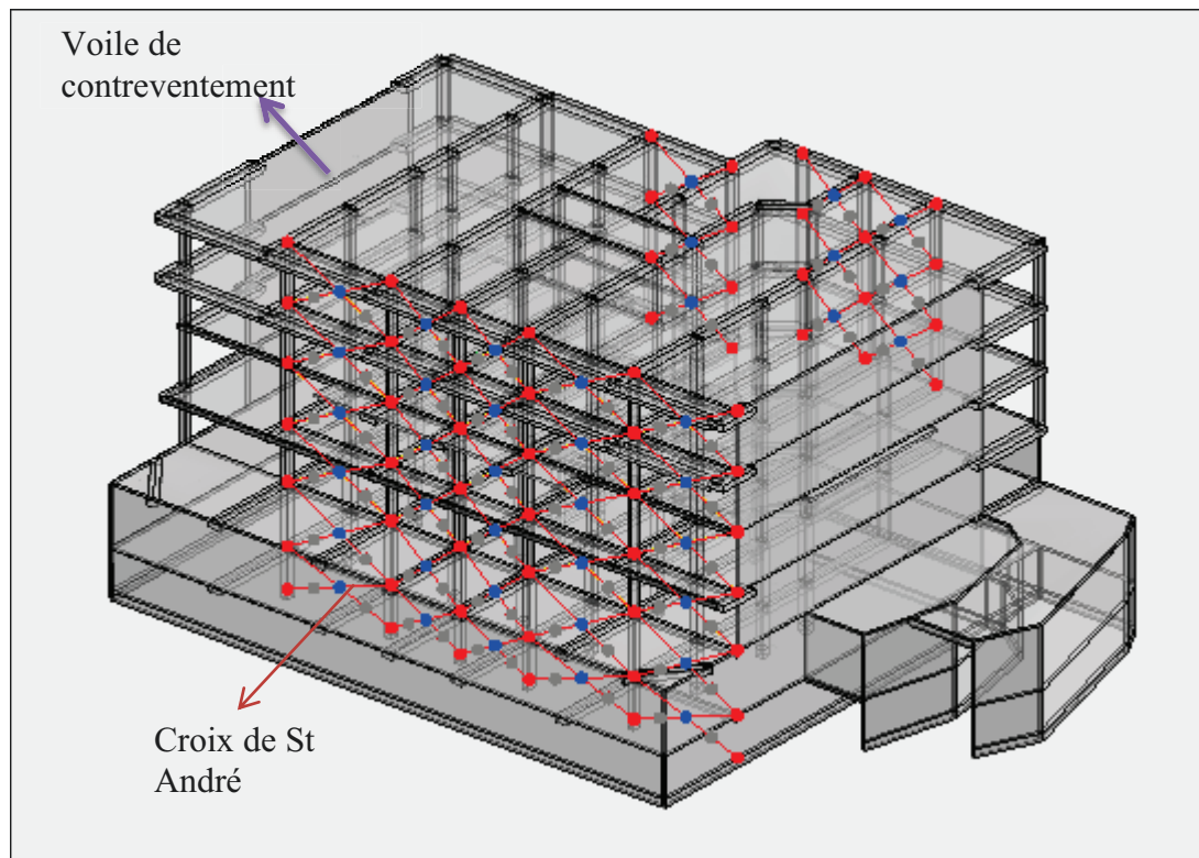
Figure 50 : Bâtiment contreventé
