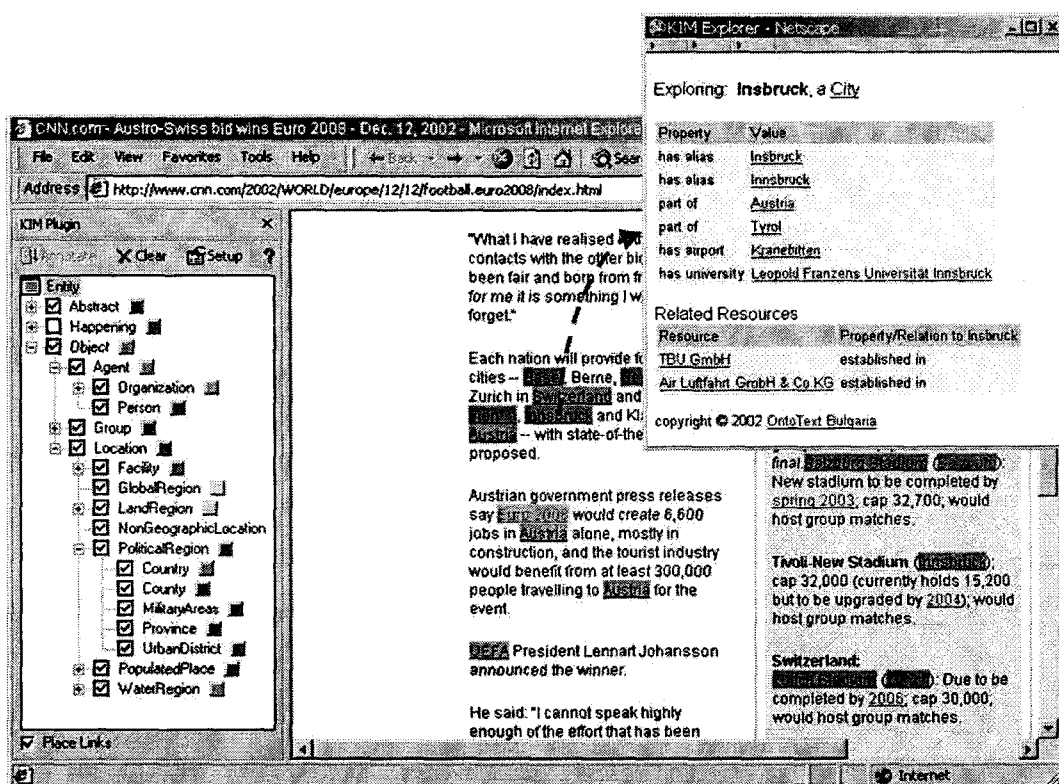
Figure 15: le plug-in KIM, et l'explorateur KIM (36)
