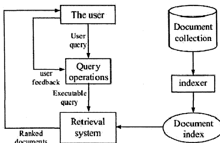
Figure 1: Un système de moteur de recherche lors d'une opération de recherche (1)
