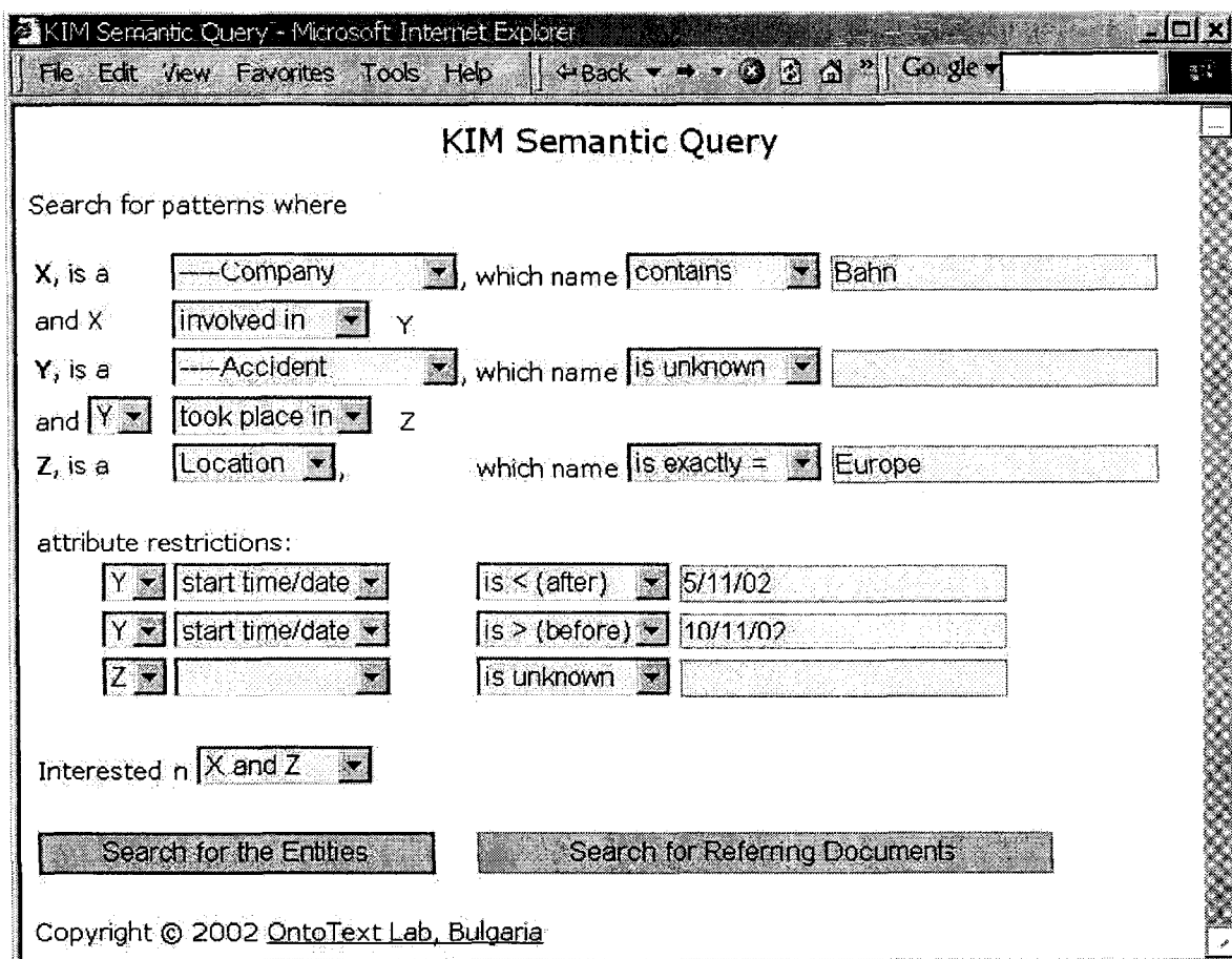
Figure 16: L'interface utilisateur d'interrogation de KIM
