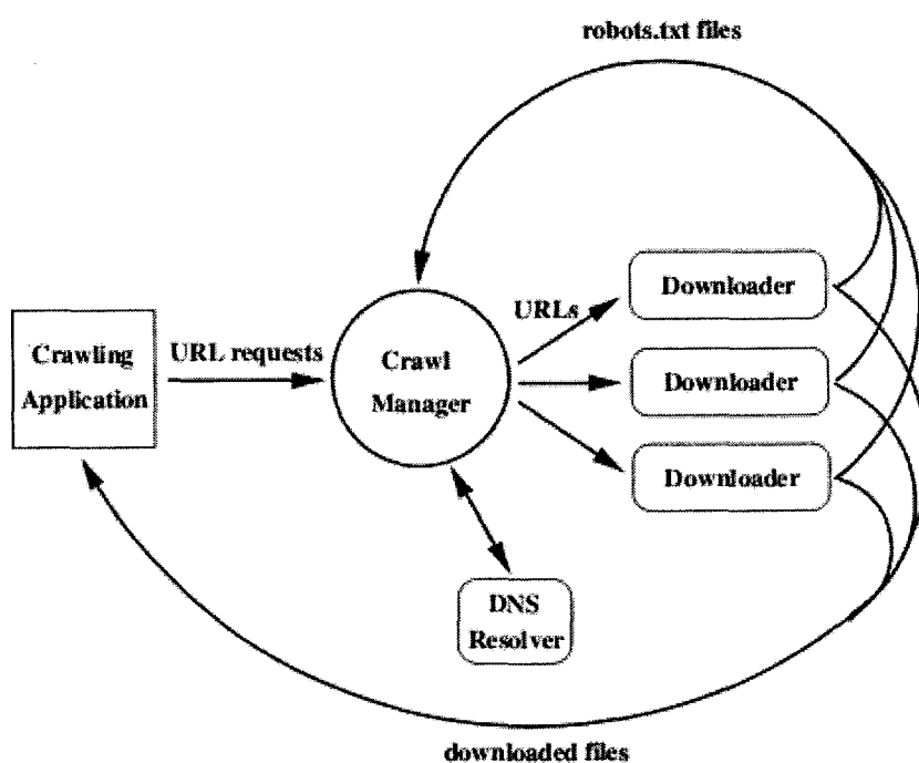
Figure 2: Un système web crawler en détail
