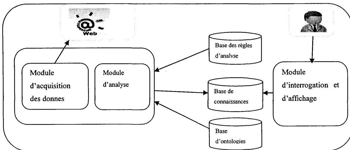
Figure 17: Architecture du Système d'analyse d'opinion
