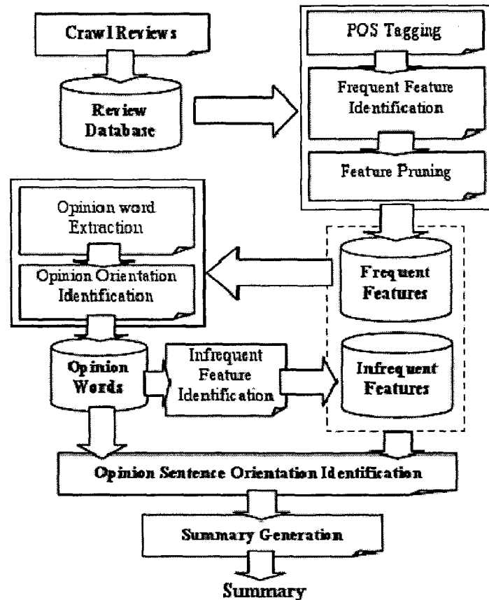
Figure 3: Architecture d'un système d'extraction d'opinion (5)
