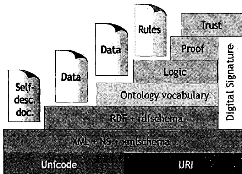
Figure 8: Architecture du web sémantique
