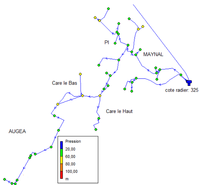
Figure 42 : Pressions à Maynal et Augea avec le nouveau réservoir plus haut
