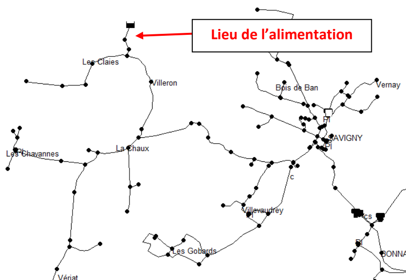
Figure 31 : Test d'alimentation du syndicat par la SAUR
