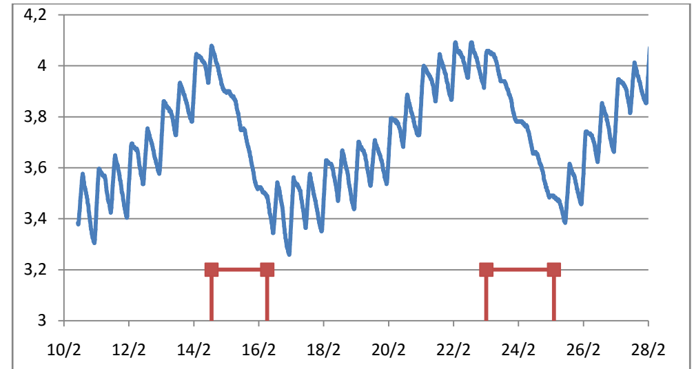
Influence de la vanne altimétrique
