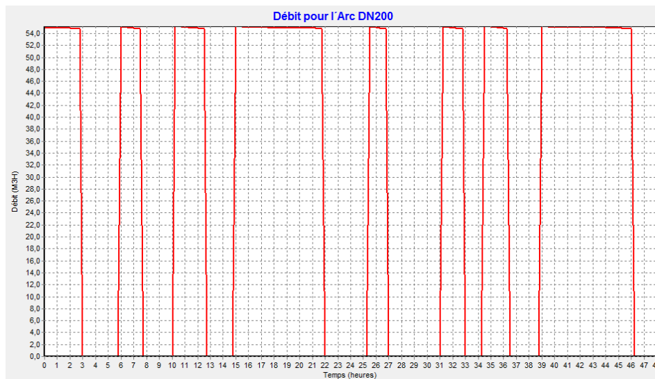
Figure 29 : Débit dans la conduite d’alimentation du réservoir de Sainte Agnès dans la situation actuelle
