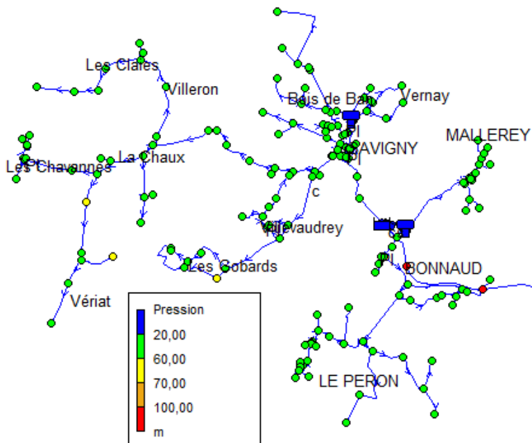
Figure 18 : Pressions pour le bas service
