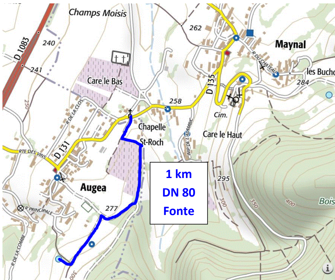
Figure 44 : Tracé de la conduite envisagée pour le raccordement d'Augea
