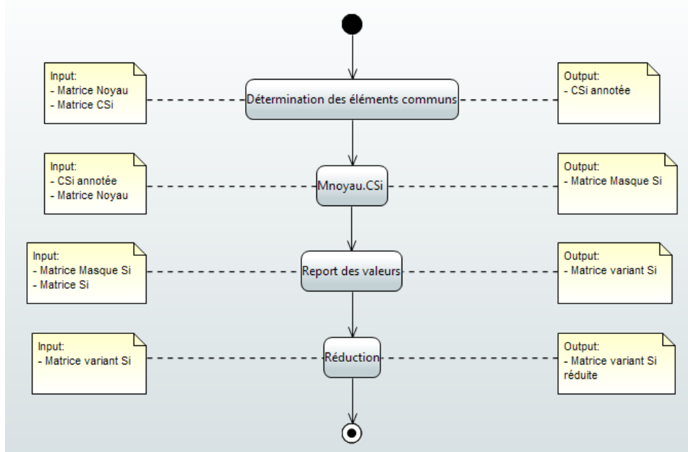
Figure 14 – Diagramme d'activité : Détermination du variant.
